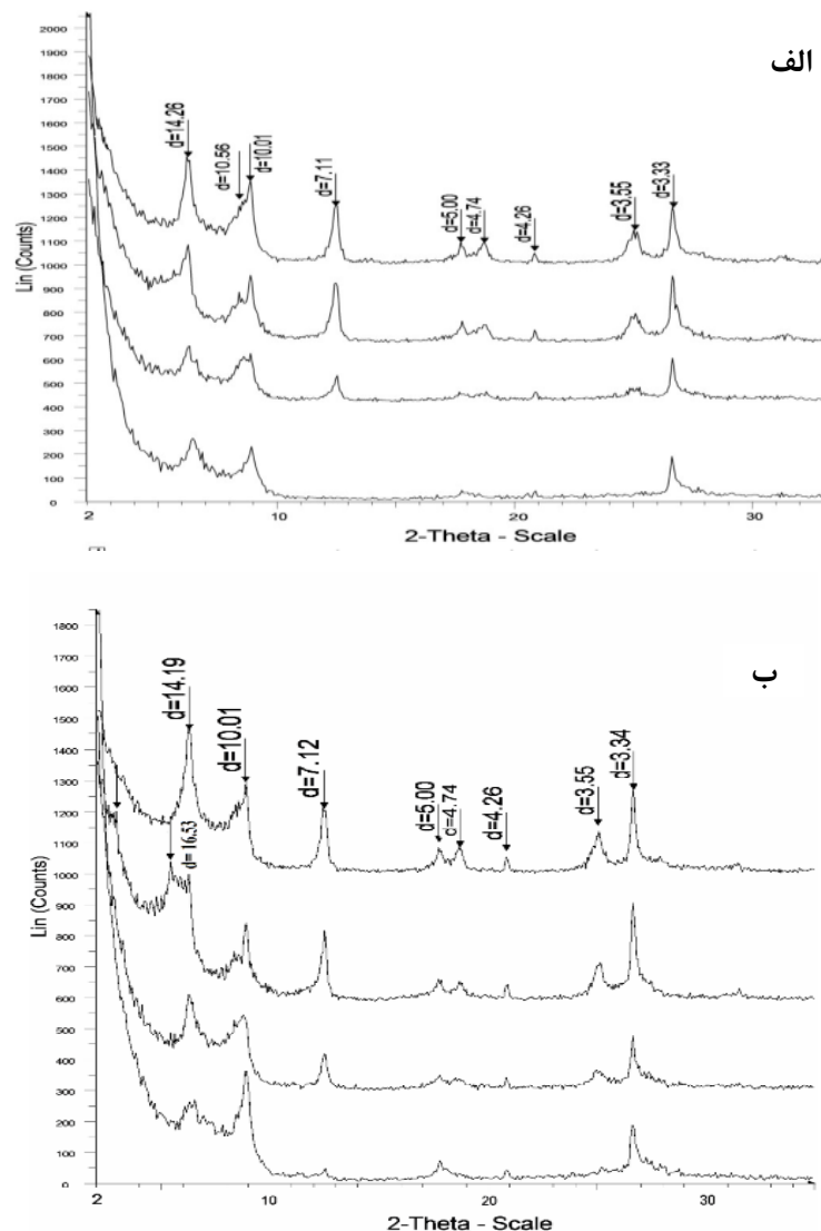
شکل ۴ الگوی XRD الف: افق Ap و ب: افق BK3 نیمرخ حفر شده در مزرعه زیر کشت تناوبی (اعداد ارائه شده بر قله‌ها فاصله بین صفحه‌ای بر حسب آنگستروم و طیف‌ها از بالا به پایین به ترتیب مربوط تیمار منیزیم، منیزیم و گلیسرول، پتاسیم و تیمار پتاسیم و گرمای ۵۵۰ درجه سانتی‌گراد هستند).
