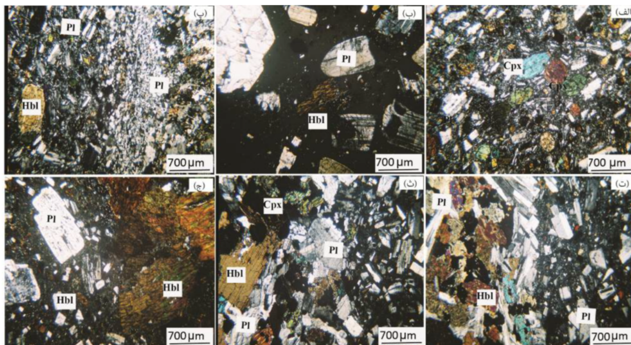
شکل ۳ (الف) بافت میکرولیتی پورفیری در سنگ میزبان آندزیت (XPL)، (ب) بافت هیالوپورفیری در سنگ میزبان (XPL)، (پ) مرز میانبار همزاد با سنگ میزبان (XPL)، (ت، ث) مرز میانبار دیوریتی با آندزیت میزبان (XPL)، (ج) مرز میانبار انباشتی غنی از آمفیبول با آندزیت میزبان (XPL).
