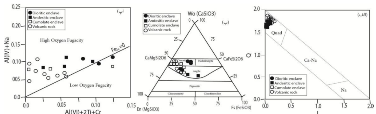
شکل ۴ الف) ترکیب کلینوپیروکسن در نمودار Q = Ca+Mg+Fe (II) نسبت به J [۱۷]، J = 2Na و Q = Ca+Mg+Fe (II) (ب) رده بندی پروکسن‌ها در نمودار Ca-Mg-Fe [۱۸]، (پ) نمودار تغییرات Na + Al^{IV} نسبت به Al^{VI} + 2Ti + Cr [۱۹].
