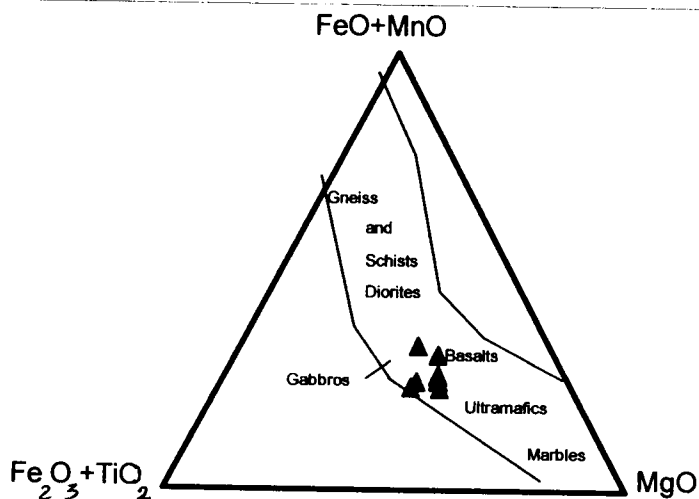
شکل ۱۱ - B نمودار تغییرات ترکیب شیمیایی فلوگوپیت‌ها و بیوتیت‌ها با نوع سنگ (نمودار کامل شده هنریچ، ۱۹۴۶ در [۵]. با توجه به این نمودار تمامی میکاهای مورد مطالعه در محدوده سنگهای گابرویی و بازالتها قرار می‌گیرند.
