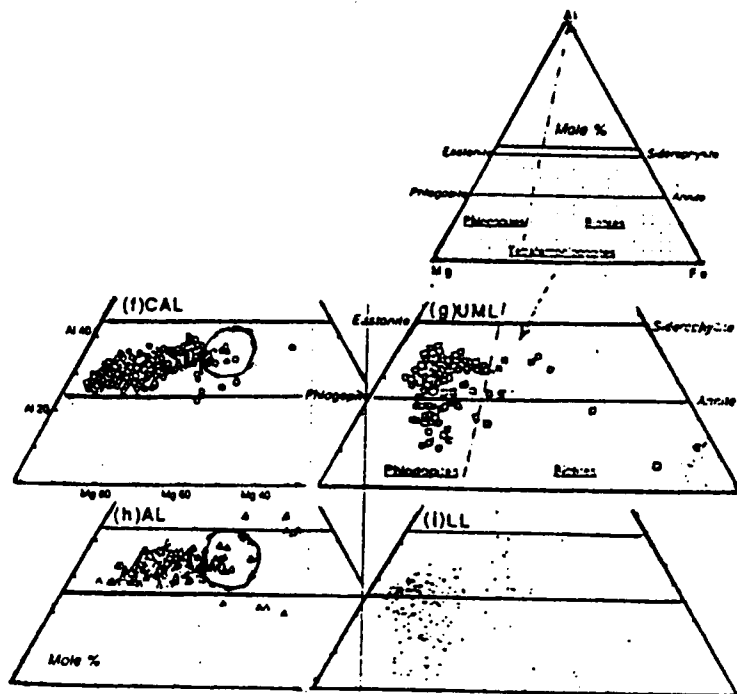
شکل ۱۰ تعیین نوع میکاها با توجه به نمودار Fe-Mg-Al، (A). مقایسه این میکاها با میکاهای انواع مختلف سنگهای لامپروفری (B) با نمودار (h) که نشانه لامپروفرهای آلکالن است مطابقت دارد، [v]. AL: آلکالی لامپروفر CAL: کالک آلکالی لامپروفر LL: لامپرویت لامپروفر UML: اولترا مافیک لامپروفر
