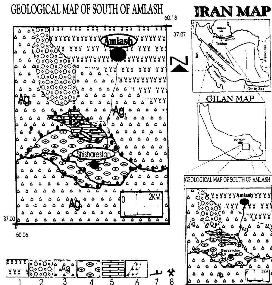
شکل ۱ نقشه زمین شناسی ناحیه مورد مطالعه.
