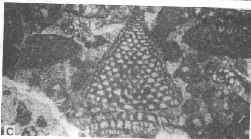
شکل ۲ نمونه‌ای از میکروفسیل‌ها در آهک‌های میزبان. دایک‌های میکادار، مبین سن آسپین هستند.
