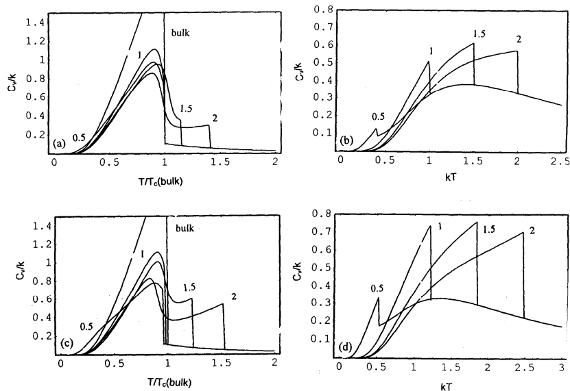
شکل ۲ گرمای ویژه بر حسب دما برای یک فیلم دوازده لایه‌ای. (الف) \Omega_s/J = 1, \Omega/J = 1, N_s = 1
