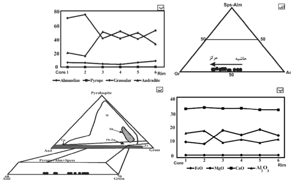
شکل ۴ الف) نمودار سه تایی (اسپسارتین + آلمانین)، (گروسولار) و (آندرادیت) [۸]. ب) نمودار منطقه‌بندی اعضای انتهایی بلور گارنت. پ) نمودار منطقه‌بندی عناصر موجود در بلور گارنت. ت) ترکیب گارنت‌های مورد بررسی در نمودار (Andradite-Grossular) برای مقایسه با گارنت‌های اسکارن [۹].
