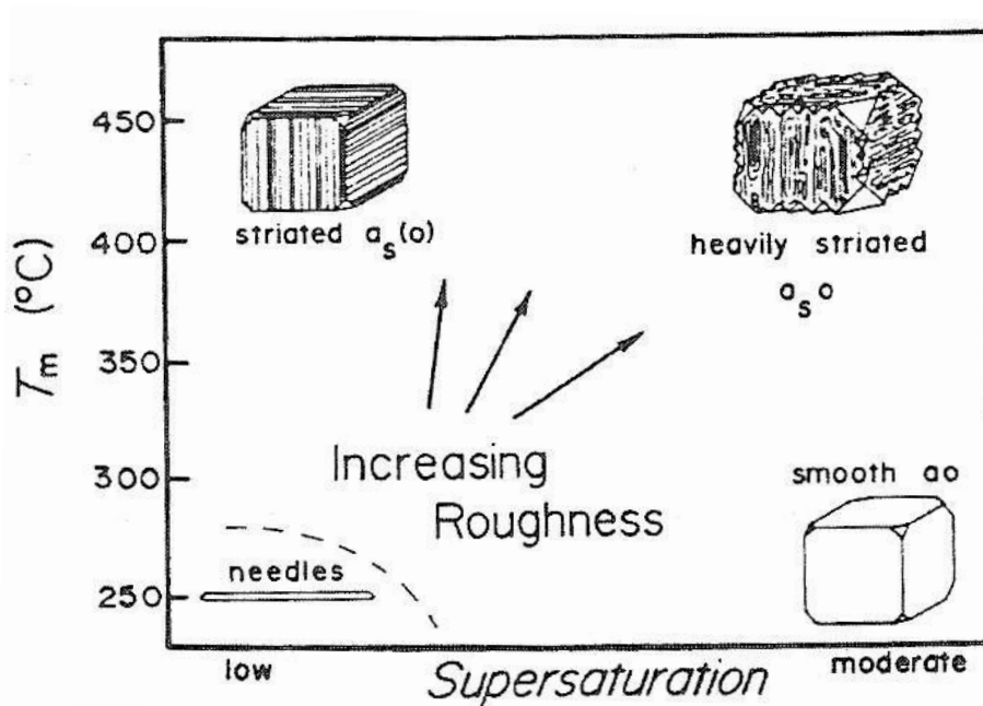
شکل ۳ اشکال مختلف رشد بلوری در کانی پیریت و در شرایط گرمایی T_m = دمای متوسط، a = (100) ، o = (111) ، شیار دار s = [6] . o = سطوح با گسترش کمتر.
