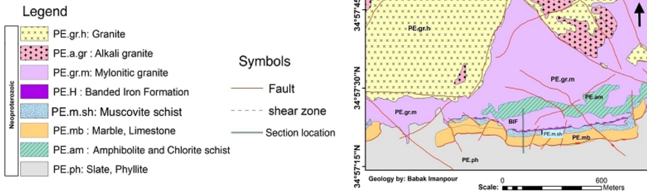
شکل ۲ نقشه زمین شناسی منطقه و موقعیت مقطع زمین شناسی منطقه‌ی ده‌زمان.
