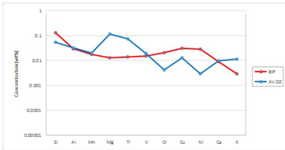
شکل ۷ نمودار عنکبوتی عناصر جزئی اکسیدهای آهن در کانسارهای آهن نواری (BIF) [۱۰] و مقایسه‌ی آن با منحنی کانسنگ هماتیتی کانسار آهن ده‌زمان.
