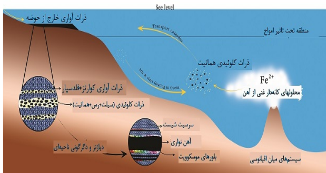
شکل ۹. ارائه‌ی مدل کانسار آهن ده‌زمان و حمل کلئیدی آهن به‌وسیله‌ی ذرات سیلت و رس آواری.
