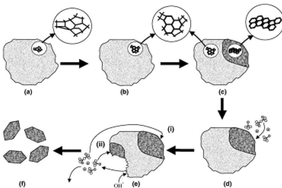
شکل ۶ طرحواره‌ای از روند پیشنهادی فلانینگ و برک [۹]. استقرار یافتن مناطق نظم یافته؛ رشد مناطق نظم یافته و تشکیل هسته‌های اولیه؛ رشد هسته‌های اولیه با کمک مواد محلول؛ رشد و گسترش یافتن مواد تازه متبلور شده؛ حل شدن بیش از پیش مواد اولیه برای پشتیبانی از یک-های در حال رشد و تبدیل تمام مواد اولیه به ماده بلورین جدید.
