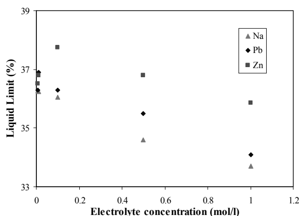
شکل ۱ تاثیر غلظت الکترولیت‌های مختلف بر حد روانی کائولینیت.
