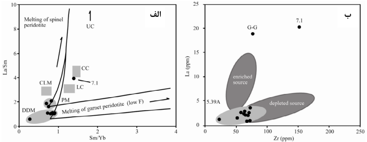
شکل ۸ نمودارهای الف) La/Sm نسبت به Sm/Yb [۲۷] و ب) Zr نسبت به La [۲۷] برای اکلوزیت‌های شاندرمن.
