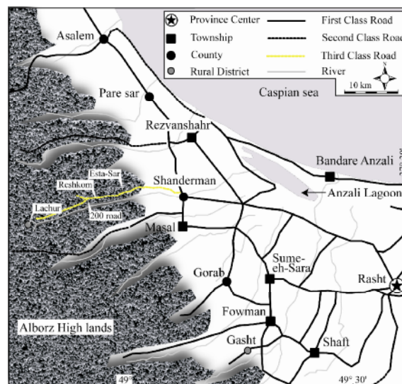
شکل ۱ موقعیت منطقه‌ی مورد بررسی (شکل بالا) و راه‌های دسترسی به آن (شکل پایین).
