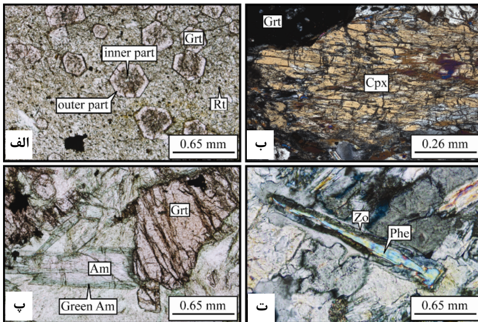
شکل ۳ تصاویر میکروسکوپی از الکلزیت‌های شاندرمن، (الف) نمایش بخش مرکزی و خارجی گارنت‌ها (PPI) (ب) کلینوپیروکسن و گارنت‌های اوج دگرگونی (XPL) (پ) آمفیبول‌های منطقه‌ای و شکستگی‌های موازی در گارنت (PPL) (ت) رشد تأخیری زوئیزیت در اطراف فنزیت (XPL). علائم اختصاری کانی‌ها از [۱۴]: گارنت: Grt، روتیل: Rt؛ کلینوپیروکسن: Cpx؛ آمفیبول: Am؛ زوئیزیت: Zo؛ فنزیت: Phe.
