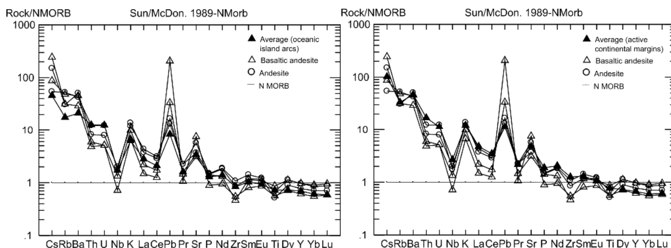
شکل ۹. مقایسه‌ی الگوهای به‌نچار شده‌ی عناصر نادر آندزیت‌های بازالتی و آندزیت‌های منطقه‌ی مورد بررسی با نمودارهای عنکبوتی میانگین جزایر قوسی و میانگین حواشی قاره‌ای فعال [۱۴].
