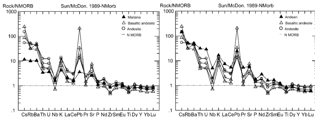
شکل ۸. مقایسه‌ی الگوهای به‌نچار شده [۳۳] عناصر نادر آندزیت‌های بازالتی و آندزیت‌های منطقه‌ی مورد بررسی با نمودارهای عنکبوتی ماریانا و آند [۱۴].
