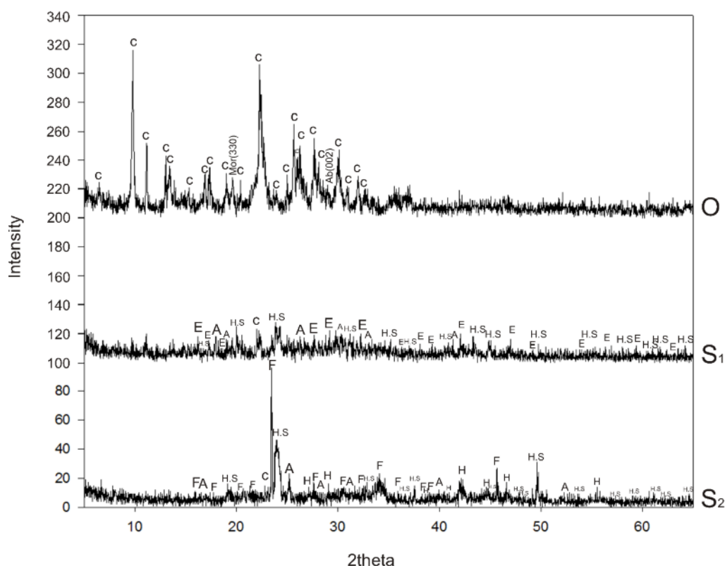
شکل ۶ نمودارهای پراش پرتو ایکس نمونه‌ی اولیه (O)، نمونه‌ی سنتزی (S 1b )، و نمونه‌ی سنتزی دوم (S 2b )، در نمودارهای مورد نظر، (C) : کلینوپتیلولیت، (Mor) : مورنیت، (Ab) : آلبیت، (E) : ادینگتونیت، (H) : هارموتوم، (F) : فوجاسیت، (A) : آنالسیم و (H.S) : هیدروسودالیت.
