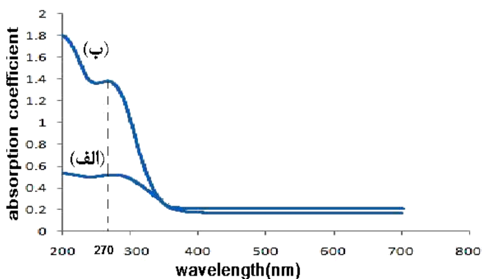
شکل ۸ بیناب جذب ناحیه دیدگان-فرابنفش برای وجه (100) از الف: بلور خالص KDP و ب: \text{KDP} + 0.01\text{ wt\% EDTA} بلور با ناخالصی \text{Al}^{3+} دارای جذب اضافی در ناحیه ۲۰۰-۳۵۰ nm با قله‌ای در ۲۷۰ nm است.
