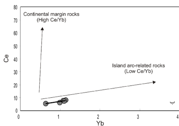
شکل ۹ الف) نمودار La نسبت La/Yb نشان می‌دهد که تحول ماگما بیشتر تحت تاثیر ذوب بخشی است. ب) تغییرات میزان Yb نسبت به Ce برای سنگ‌های گابرویی مورد بررسی. روندهای جزایر قوسی (پایین Ce/Yb ) و حاشیه‌ی قاره‌ای ( Ce/Yb بالا) از [۲۶].
