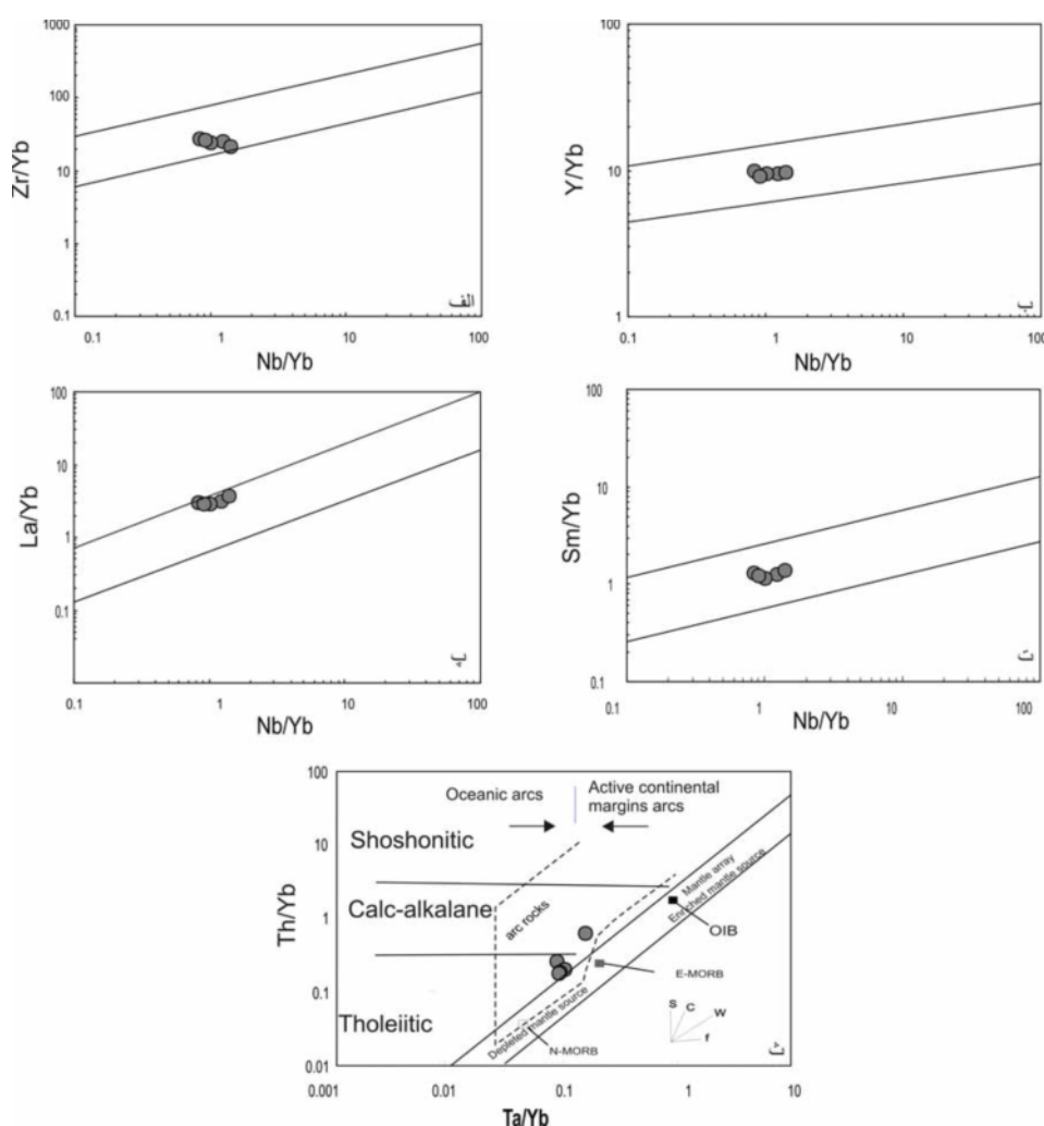
شکل ۱۱ نمودار M/Yb نسبت به Nb/Yb سنگ‌های گابرویی بغم. الف) Zr/Yb ب) Y/Yb پ) La/Yb و ت) Sm/Yb . MORB و OIB به ترتیب معرف خاستگاه گوشته جزایر اقیانوسی و پشته‌ی میان اقیانوسی است. آرایه گوشته‌ای (آرایه OIB-MORB) اقتباس از [۵۱]. ث) نمودار Th/Yb بر حسب Ta/Yb با آرایه‌ی گوشته‌ای اقتباس از Pearce (1983) که نشان‌دهنده‌ی نقش اجزای درگیر در فرورانش، c آلودگی پوسته‌ای، w غنی‌شدگی درون صفحه‌ای و f تبلور بخشی.
