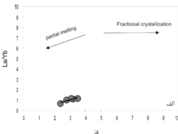
شکل ۹ الف) نمودار La نسبت La/Yb نشان می‌دهد که تحول ماگما بیشتر تحت تاثیر ذوب بخشی است. ب) تغییرات میزان Yb نسبت به Ce برای سنگ‌های گابرویی مورد بررسی. روندهای جزایر قوسی (پایین Ce/Yb ) و حاشیه‌ی قاره‌ای ( Ce/Yb بالا) از [۲۶].
