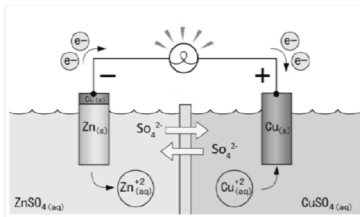
شکل ۲ نمایی از یک سلول گالوانی.
