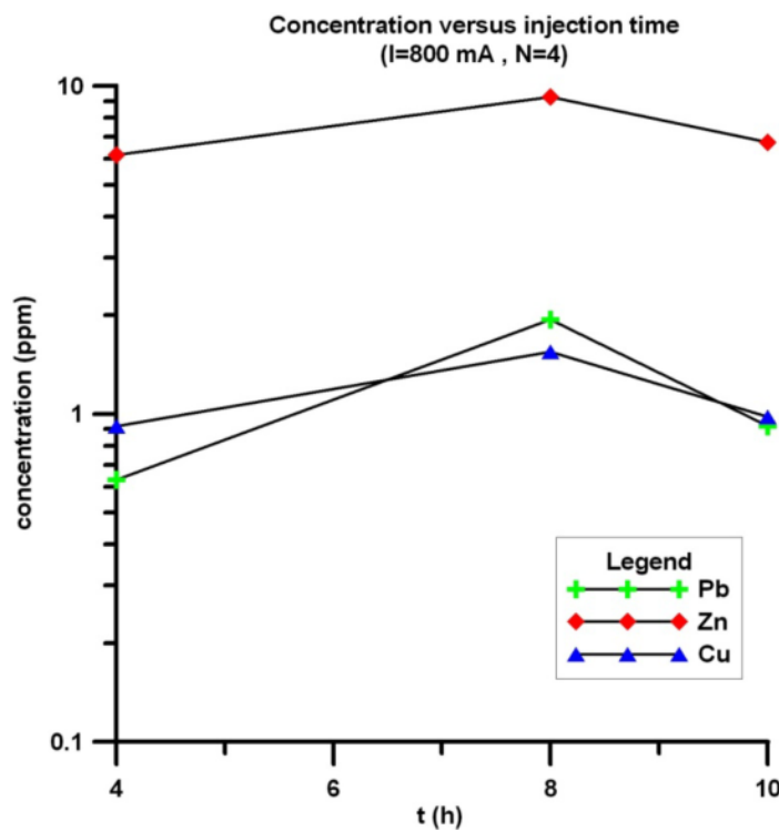
شکل ۱۱ تغییرات غلظت عناصر نسبت به زمان تزریق جریان (در شرایط ثابت نرمالیته اسید مصرفی ۴ و شدت جریان تزریقی ۸۰۰mA).
