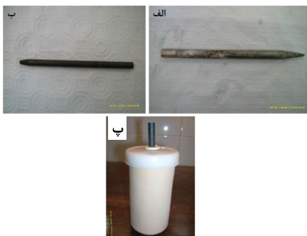
شکل ۶ الف. الکتروود فولادی مورد استفاده در آند و خوردگی سطح آن ناشی از اسیدی شدن محیط آند، ب. میله‌ی گرافیتی مورد استفاده در کاتد، پ. الکتروود کاتدی شامل کوزه سفالی همراه با میله‌ی گرافیتی که با درپوش مخصوص در مرکز کوزه قرار گرفته و هنگام قرارگیری در درون خاک با الکتروولیت (اسید نیتریک) پر می‌شود.
