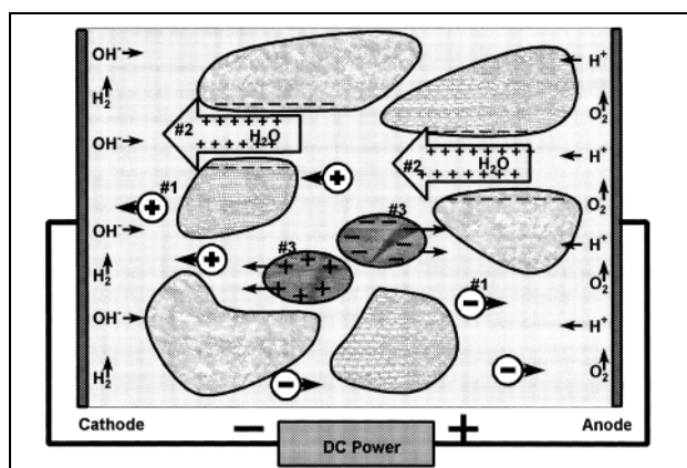
شکل ۳ نقش آب و فرایندهای مهم در الکتروژئوشیمی (آزاد شدن گاز هیدروژن و ایجاد یون هیدروکسید در کاتد و آزاد شدن گاز اکسیژن و اسیدی شدن آنده) [۵].
