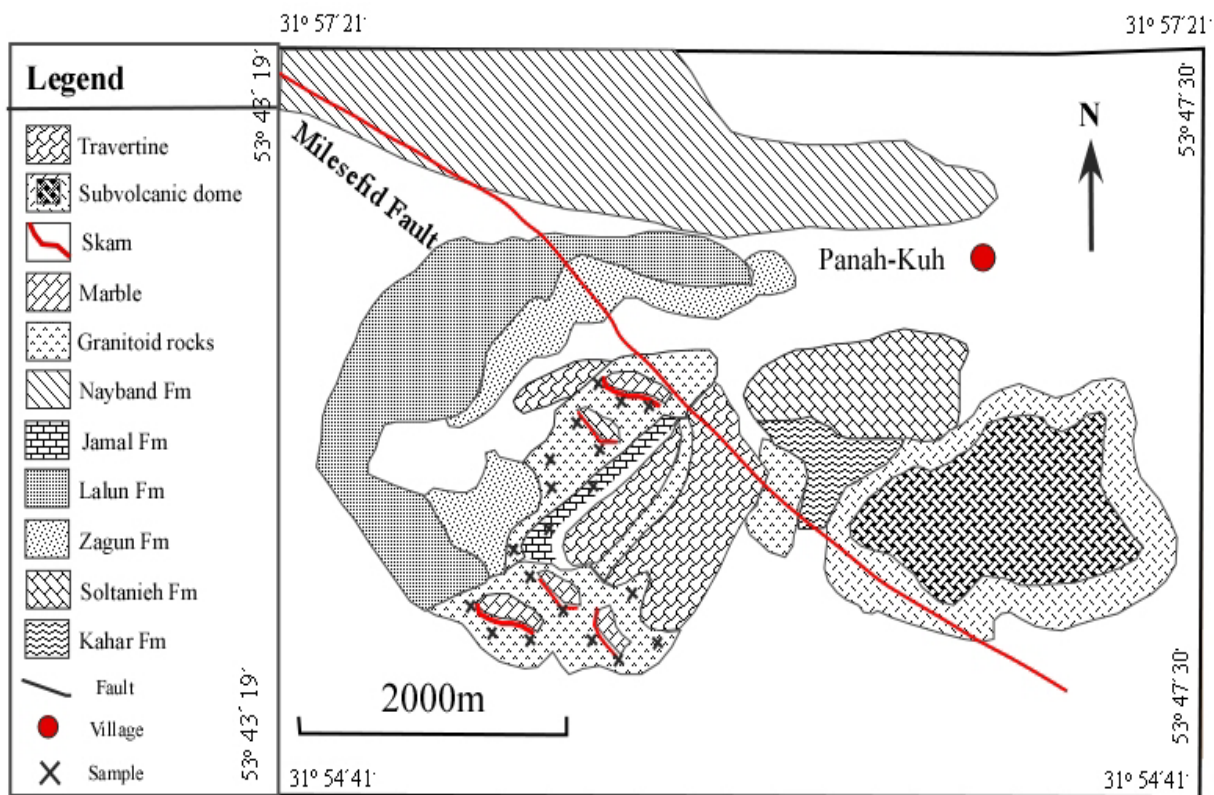
شکل ۱ نقشه‌ی زمین‌شناسی منطقه پناهکوه واقع در غرب استان یزد بر اساس مطالعات صحرایی و استفاده از عکس‌های هوایی (اقتباس از نقشه زمین‌شناسی ۱:۱۰۰۰۰۰ خضراًباد با تغییرات).
