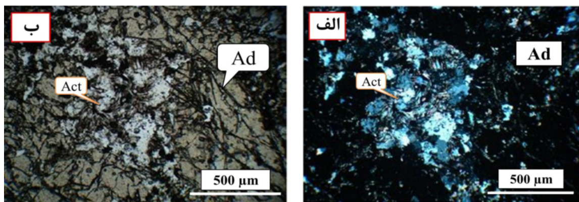
شکل ۱۰ قرار گرفتن اکتینولیت به صورت مستقل و در همراهی با کوارتز در فضای بین آندرادیت‌ها (الف: نیکل عمود ب: نیکل موازی).
