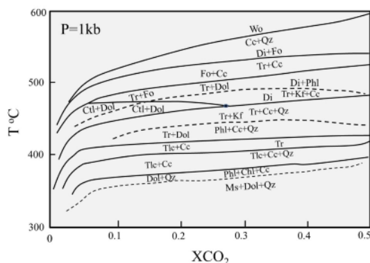
شکل ۱۳ نمودار روابط فاز T-X_{CO_2} در سامانه Al-K-Ca-Mg-Si-H-C-O [۱۲].
