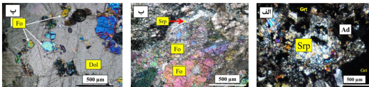
شکل ۷ الف جانشینی کامل اولیون با سرپانتین و تشکیل شبریخت حاصل از آن ب: سرپانتینی شدن اولیون و تشکیل بافت شبکه‌ای حاصل از آن در اسکارن منیزیمی. پ: درشت بلورهای اولیون سالم با پیرامون گرد شده (Resorbed) در اسکارن منیزیمی.
