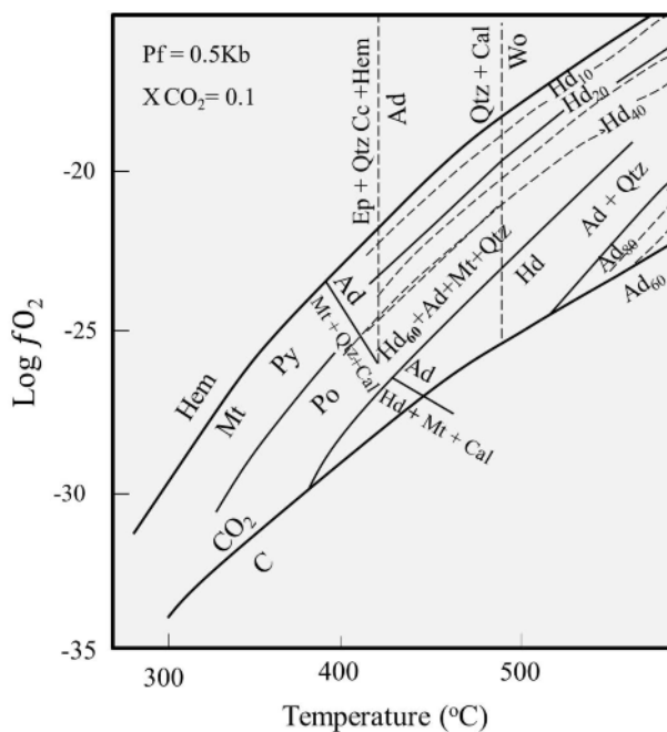
شکل ۱۲ نمودار روابط فاز T-log fO 2 در سامانه Ca-Fe-Si-C-O-H [۱۱].
