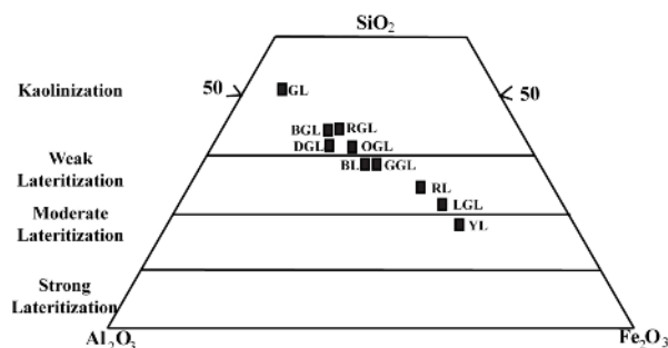
شکل ۷ نمودار ۳ متغیره ی \text{Al}_2\text{O}_3\text{-Fe}_2\text{O}_3\text{-SiO}_2 [۳۸] که شدت فرایند لاتریتی شدن در واحدهای مختلف نهشته‌ی زان را نشان می‌دهد.
