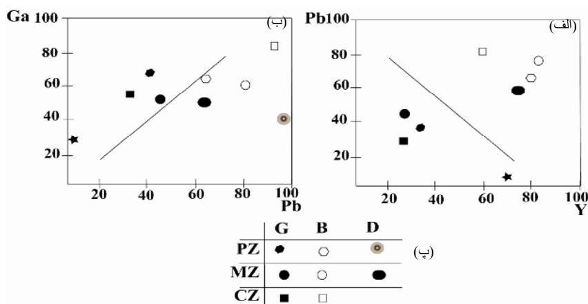
شکل ۹ الف و ب) به ترتیب نمودارهای دو متغیره ی عناصر کمیاب \text{Pb-Y} و \text{Ga-Pb} در لاتریت‌هایی با سنین و فرم‌های مختلف کانی‌های آلومینیم‌دار [۳۹]. در نمودارهای الف و ب یافته‌های لاتریتی زان با علامت ستاره نشان داده شدند و پ) علائم اختصاصی کانی‌های مختلف آلومینیم‌دار در دوران‌های مختلف زمین شناسی، در این شکل G - گیسیت، B - بوهمیت، D - دیاسپور، PZ - پالئوزویک، MZ - مزوزویک و CZ - سنوزویک.
