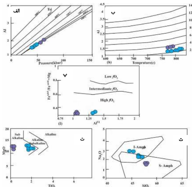
شکل ۷ ترسیم داده‌های آمفیبول توده‌های غرب تفت: در نمودار الف) فشار برحسب کیلو بار در مقابل Al^{IV} [۱۶] و محدوده دمایی تشکیل آمفیبول، ب) نمودار دما برحسب درجه سانتی‌گراد در مقابل Al^{IV} [۱۶]، پ) نمودار Al^{IV} در مقابل Fe^{T+Mg}/Fe^{T+Mg} [۱۲]، ت) جایگاه تکتونیکی آمفیبول‌های مورد مطالعه [۲۱]، ث) موقعیت ترکیب شیمیایی آمفیبول‌ها در نمودار [۲۲] (I-Amph): آمفیبول درون صفحه‌ای، (S-Amph): آمفیبول وابسته به مناطق فرورانش.
