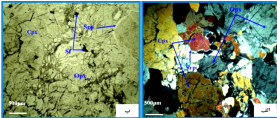
شکل ۷ کانی‌های سولفیدی (Sf)، ارتوپیروکسن (Opx) و کلینوپیروکسن (Cpx) در سنگ‌های فاریاب (Srp=سرپانتین) (الف) نور XPL و (ب) نور PPL.
