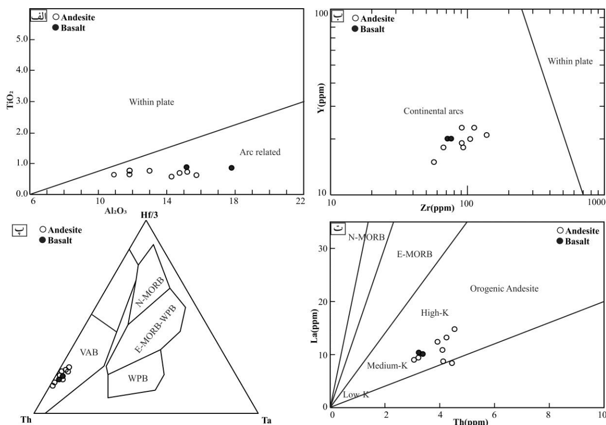
شکل ۸ نمودارهای زمین شیمیایی تعیین محیط زمین ساختی سنگ‌های آتشفشانی کوه بندسیاه (شمال غرب انارک): (الف) نمودار \text{TiO}_2 - \text{Al}_2\text{O}_3 برای آندزیت (○) و بازالت (●)، (ب) نمودار Y- Zr (۵۷)، (پ) نمودار مثلی \text{Hf}/3 - Th- Ta (۵۵) و (ت) نمودار La- Th برای تفکیک آندزیت‌های کوهزایی از سایر آندزیت‌ها [۵۶].
