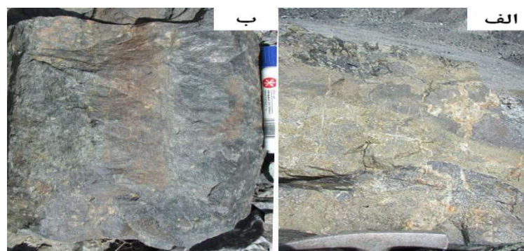
شکل ۹ الف) پیریت رگه‌ای که مگنتیت را قطع کرده و نشان‌دهنده روزادی بودن آن است، ب) پیریت به صورت انتشاری روی مگنتیت قرار دارد و بخشی از مگنتیت که به هماتیت تبدیل شده است.
