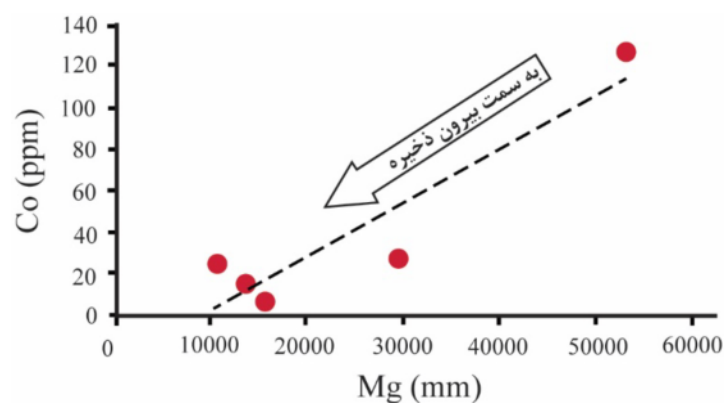
شکل ۹ تغییرات کاهش غلظت Co و Mg نمونه‌های مگنتیت از مرحله پیش‌رونده (رگچه‌ای) تا مرحله پس‌رونده (به‌مراه کانی‌های سولفیدی) در اسکارن علم‌کندی.
