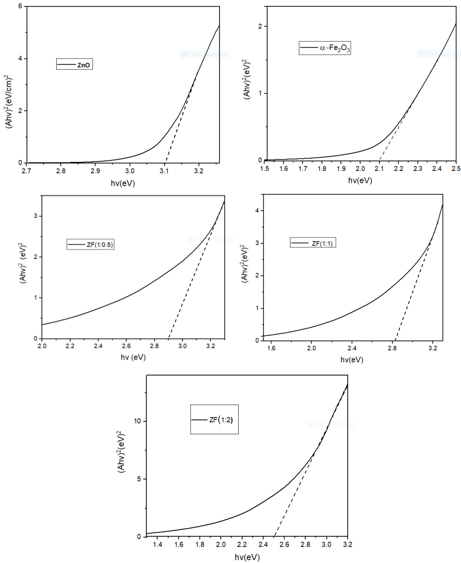
شکل ۵ نمودار (Ahv)^2 نسبت به hv برای محاسبه گاف نوری مستقیم نمونه‌ها.
