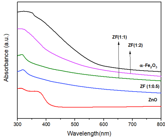
شکل ۴ طیف‌های جذب نمونه‌های ZnO، \alpha\text{-Fe}_2\text{O}_3 و نانوکامپوزیت‌های با درصد‌های وزنی مختلف \text{ZnO}/\text{Fe}_2\text{O}_3
