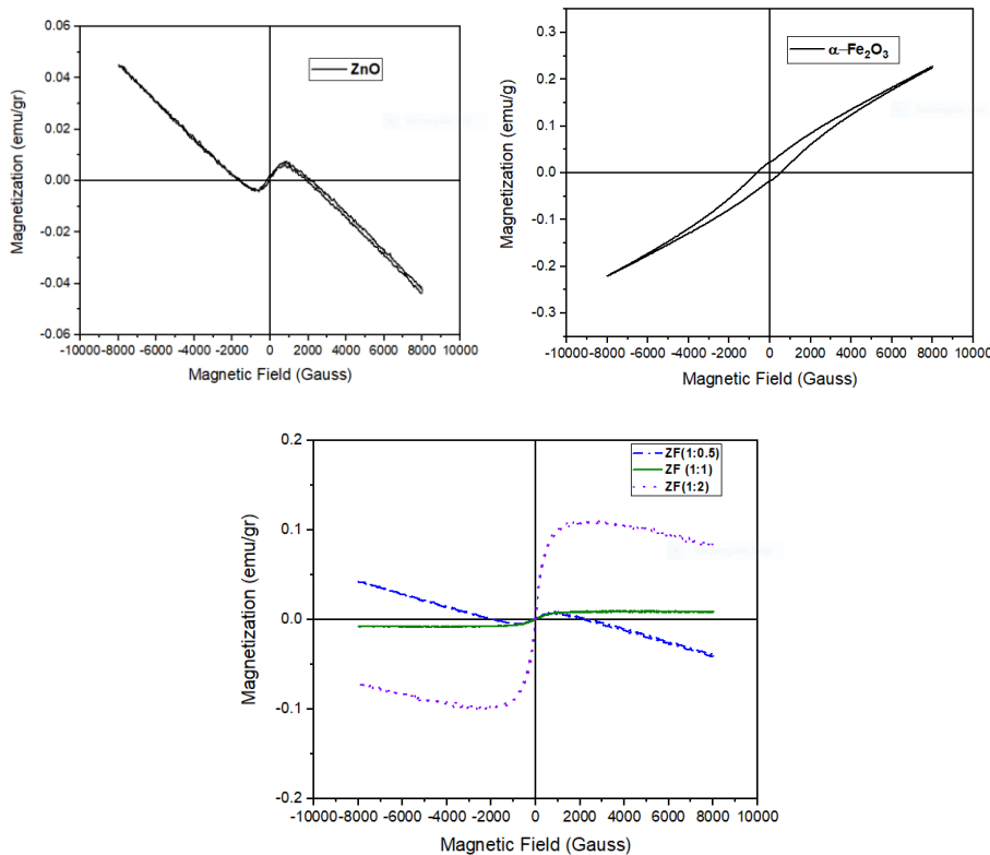
شکل ۷ منحنی‌های پسماند مغناطیسی نمونه‌های \alpha\text{-Fe}_2\text{O}_3 , ZnO و نانوکامپوزیت‌های ZnO/Fe 2 O 3
