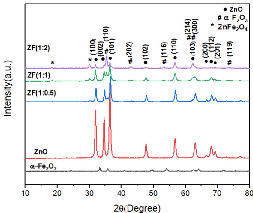
شکل ۱ الگوهای XRD نمونه‌های \alpha\text{-Fe}_2\text{O}_3 ، ZnO و نانوکامپوزیت‌های \text{ZF}(1:0.5) ، \text{ZF}(1:1) و \text{ZF}(1:2)
