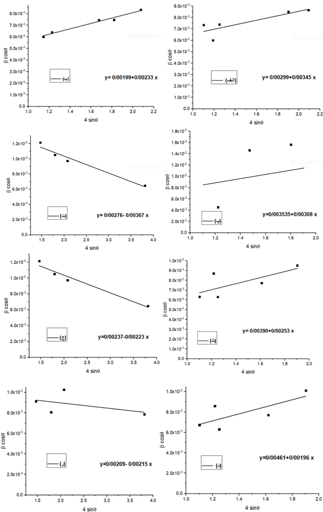
شکل ۲ نمودارهای ویلیامسون-هال رسم شده برای نمونه‌های (الف) ZnO خالص، (ب) \alpha\text{-Fe}_2\text{O}_3 خالص، (پ) و (ت) نانوکامپوزیت‌های (۵) : ۰:۰ ZF(۱)، (ث) و (ج) ZF(۱:۱)، (چ) و (ح) ZF(۱:۲)
