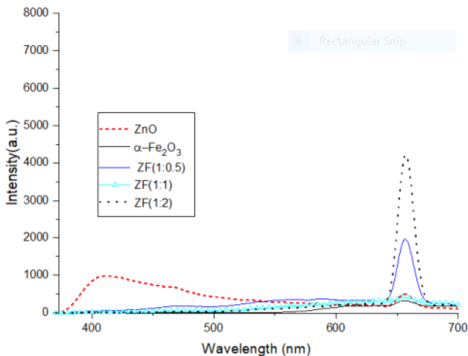
شکل ۶ طیف‌های نورتایی نمونه‌های \text{ZnO}/\text{Fe}_2\text{O}_3 ، \alpha\text{-Fe}_2\text{O}_3 و \text{ZnO}/\text{Fe}_2\text{O}_3 با درصد‌های وزنی مختلف. شکل ضمیمه گستره طول موجی ۴۰۰-۶۵۰ nm برای کامپوزیت‌ها را نشان می‌دهد.
