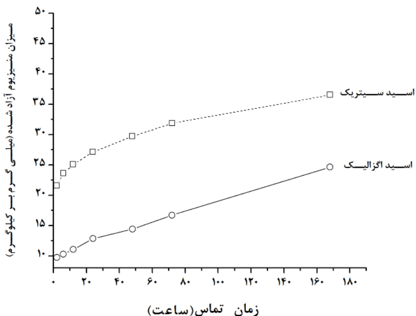
شکل ۴ تاثیر زمان تماس بین کانی واسیدهای آلی سیتریک و اگزالیک بر رهاسازی منیزیم از کانی سیپولیت.
