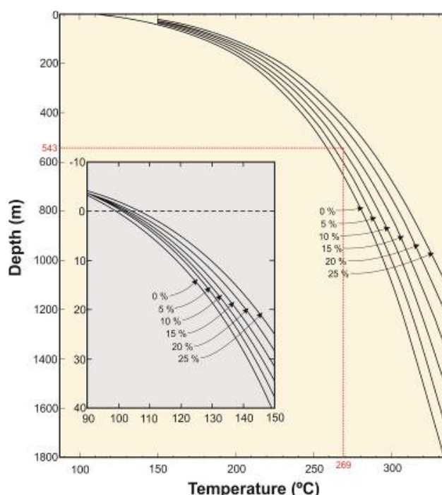
شکل ۱۲ منحنی‌های نقطه جوش مایع و شورابهایی با ترکیب ثابت. نقطه جوش مایع در فشار ۱۰۱۳ بار (۱/۰ اتمسفر) است که معادل فشار جو در سطح دریا است [۲۷].
