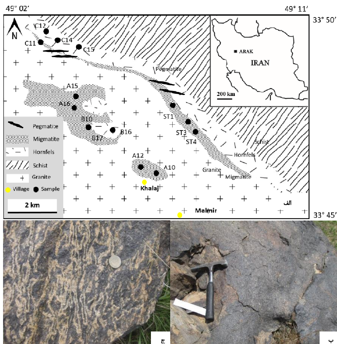
شکل ۱ الف) موقعیت جغرافیایی منطقه مورد بررسی اراک، ایران، ۲۵ کیلومتری بروجرد در منطقه بین غره‌دش و غره‌تپه، ب) رخنمون هورنفلس و پ) رخنمون میگماتیت‌ها.
