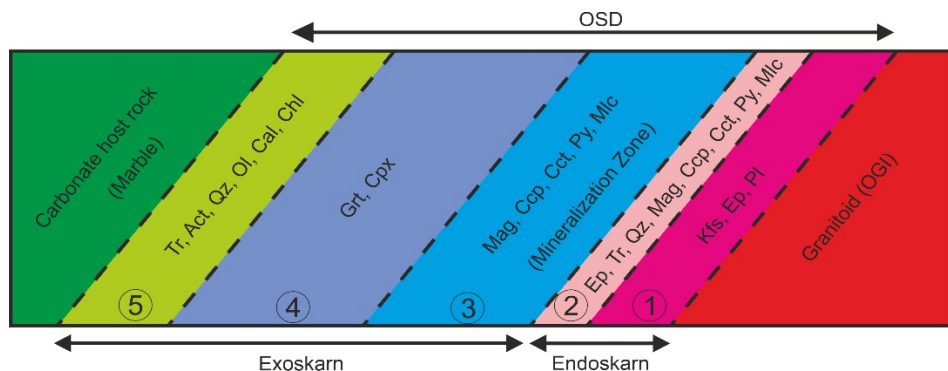
شکل ۲ موقعیت منطقه بندی درون اسکارن و برون اسکارن نسبت به توده نفوذی و سنگ میزبان کربناتی (نشانه های اختصاری از [A]).
