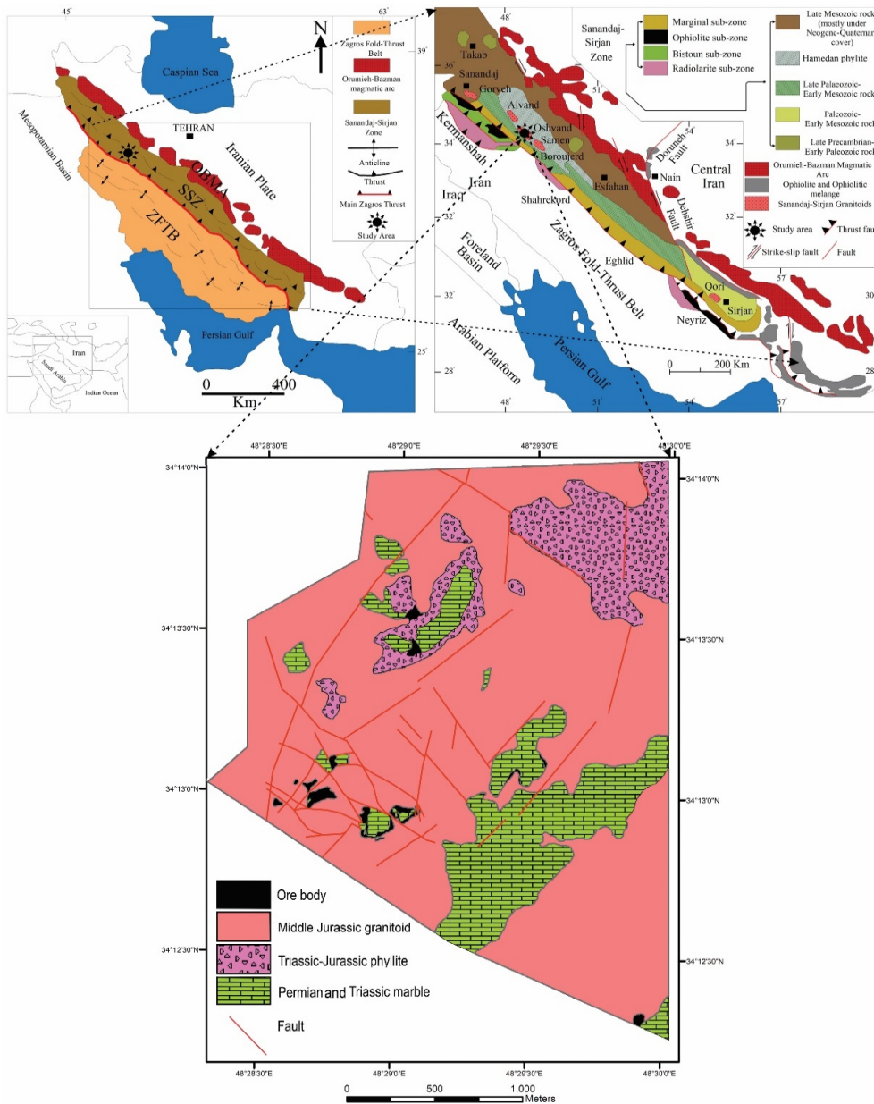
شکل ۱ نقشه زمین‌شناسی ساده شده منطقه مورد بررسی و موقعیت آن در پهناوندی ساختاری ایران برگرفته از مرجع [۱] با تغییرات.
