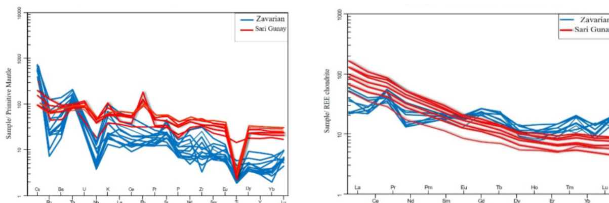
شکل ۹ الگوی توزیع عناصر نادر خاکی عادی سازی شده (normalize) نسبت به کندریت در منطقه زواریان و ساری گونای [۲۹].
