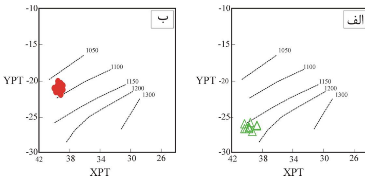
شکل ۹ نمودارهای YPT نسبت به XPT [۳۳] برای تعیین دمای تبلور الف) کلینوپیروکسن و ب) ارتوپیروکسن منطقه زولسک.
