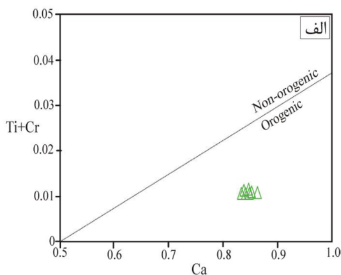
شکل ۸ الف) نمودار Ti+Cr نسبت به Ca [۱۴] و ب) نمودار F1 نسبت به F2 [۱۳] برای تعیین محیط زمین ساختی گدازه‌های آندزیتی منطقه زولسک بر اساس ترکیب کلینوپیروکسن: (OFB): بازالت‌های بستر اقیانوس، WPT: بازالت‌های تولیتی میان صفحه‌ای، WPA: بازالت‌های قلیایی میان صفحه‌ای و VAB: بازالت‌های کمان آتشفشان).
