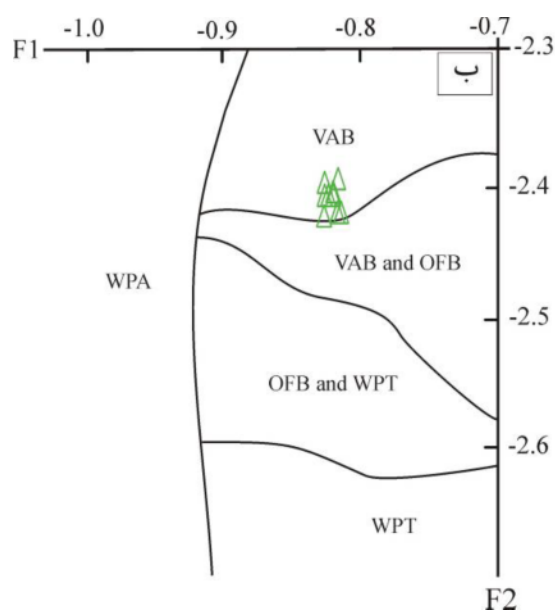
شکل ۸ الف) نمودار Ti+Cr نسبت به Ca [۱۴] و ب) نمودار F1 نسبت به F2 [۱۳] برای تعیین محیط زمین ساختی گدازه‌های آندزیتی منطقه زولسک بر اساس ترکیب کلینوپیروکسن: (OFB): بازالت‌های بستر اقیانوس، WPT: بازالت‌های تولیتی میان صفحه‌ای، WPA: بازالت‌های قلیایی میان صفحه‌ای و VAB: بازالت‌های کمان آتشفشان).
