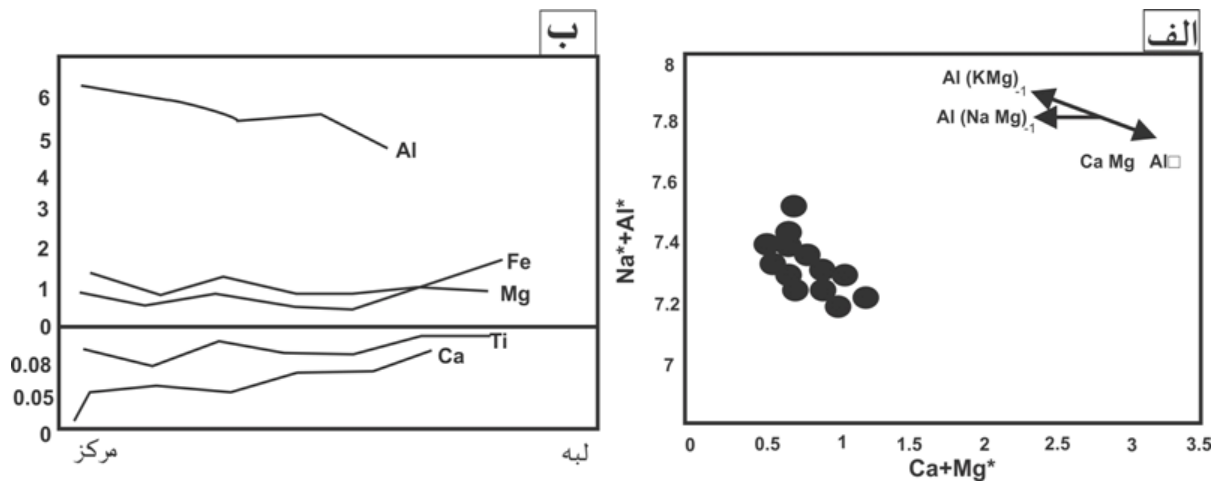
شکل ۷: الف) همبستگی وارون Ca+Mg^* در برابر Na^*+Al^* (ب) تغییرات منطقه‌بندی شیمیایی در تورمالین منطقه‌ی مورد بررسی. Mg^* = Mg + Fe + Mn + 2Li - Ti , Na^* = Na + K , Al^* = Al + Fe_3 + 2Ti - Li
