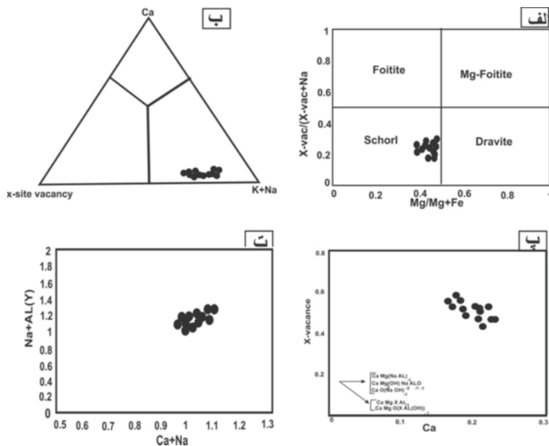
شکل ۵: الف) ترکیب تورمالین گرهکی در گستره شورلیت - دراویت به سمت شورلیت (ب) نمودار مثلثی (Na+K) و Ca و X-site vacancy و قرارگیری تورمالین گرهکی در محل قلیایی. (پ) نمودار نشان دهنده‌ی جانشینی بیشتر در تورمالین. (ت) نمودار برای تعیین نوع جانشینی موجود در تورمالین.
