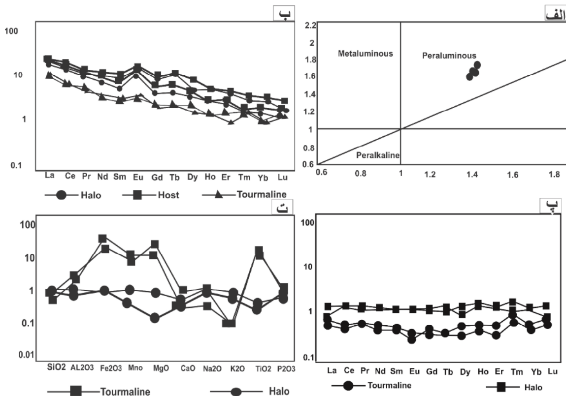
شکل ۴ الف) نمودار تعیین شاخص اشباع از آلومینیم Al/NCK نسبت به Al/NK (ب) نمودار عنکبوتی بهنجار شده‌ی REE های سنگ میزبان و هاله‌ی لوکوکرات و تورمالین بر اساس کندریت ها [۳۳]. پ) نمودار بهنجار شده‌ی REE های هاله‌ی لوکوکرات وکانی تورمالین نسبت به سنگ میزبان. ت) نمودار بهنجار شده‌ی عناصر اصلی هاله لوکوکرات و تورمالین بر اساس سنگ میزبان.
