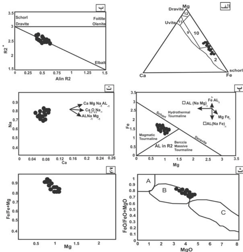
شکل ۶: الف) موقعیت تورمالین‌های گرھکی در نمودار مثلثی Ca-Fe-Mg: ۲: گرانیتوئیدهای فقیر از لیتیم، پگماتیت‌ها و آپلیت‌ها وابسته به آن‌ها. ۹: سنگ‌های کالکوسیلیکاته، متاپسامیت‌ها و متاپلیت‌های غنی از Ca. ۱۰: سنگ‌های کوارتز-تورمالین، متاپسامیت‌ها و متاپلیت‌های فقیر از Ca. ۱۱: متاکربنات‌ها ۱۲: اولترامافیک‌های دگرگون شده. ب) نمودار R2* نسبت به Al in R2. R2^* = Fe + Mg + Mn + Al , R2 = Al + 1.33 + Si - 12 . ج) نمودار Fe در برابر Mg و موقعیت تورمالین‌های گرھکی در آن. ت) قرارگیری نمونه‌ها در نمودار Ca در برابر Na (ث) نمودار FeO/(FeO+MgO) در برابر MgO که نشان دهنده قرارگیری تورمالین‌ها در موقعیت B است. ج) نمودار Fe/(Fe+Mg) در برابر Mg که نشان دهنده تمایل تورمالین‌ها در جهت Fe بیشتر است.
