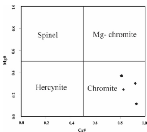
شکل ۷ موقعیت کرومیت‌های منطقه در نمودار Cr^{\#}-Mg^{\#} [۲۱].
