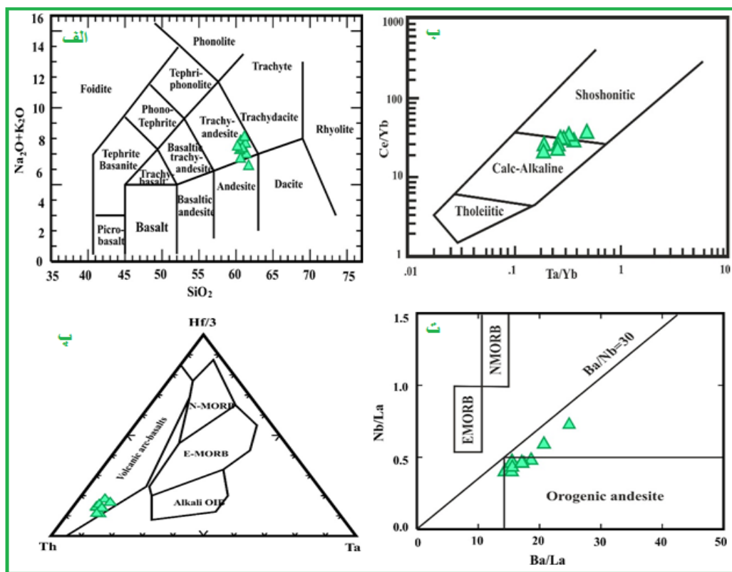
شکل ۵ الف) نمودار مجموع قلیاییها (Na 2 O+K 2 O) نسبت به SiO 2 [۱۳] ب) نمودار Ce/Yb نسبت به Ta/Yb [۱۴]، پ) نمودار Th-Hf/3-Ta [۱۶]، ت) نمودار Nb/La نسبت به Ba/La [۱۷، ۱۸].
