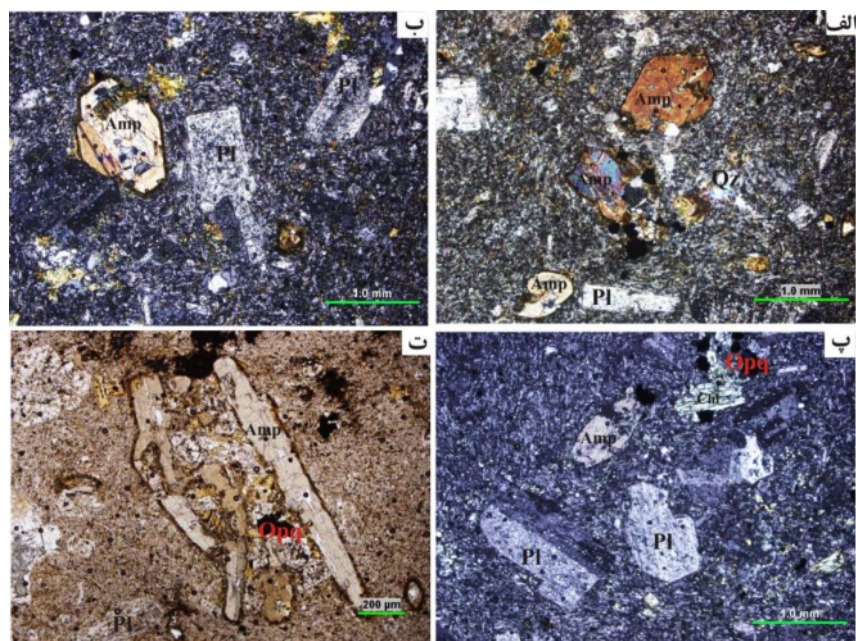
شکل ۳ تصاویر میکروسکوپی از الف و ب) بافت پورفیری با درشت بلورهای آمفیبول و پلاژیوکلاز (در نور قطبیده متقاطع، XPL)، ب) بافت غربالی و خوردگی خلیجی در پلاژیوکلازها (XPL)، ت) کانی‌های آمفیبول که در مقاطع طولی به صورت رشته ای هستند، به همراه کانی‌های پلاژیوکلاز (در نور قطبیده، صفحه‌ای PPL). نشانه‌های اختصاری برگرفته از مرجع [۱۲] هستند.
