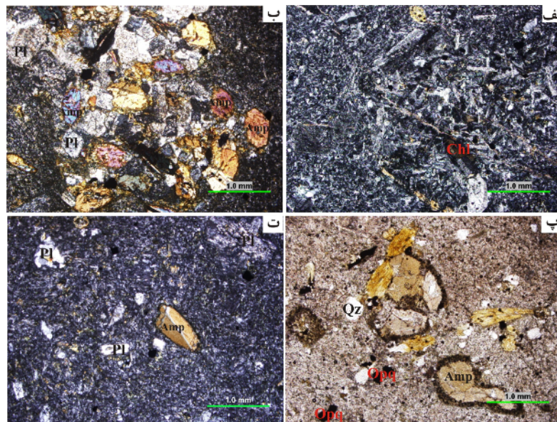
شکل ۴ تصاویر میکروسکوپی از الف) بافت ریزسنگی در سنگ‌های منطقه مورد بررسی (XPL)، ب) بافت گلوپروپرفیری ناشی از انباشت کانی‌های آمفیبول و پلاژیوکلاز (XPL)، پ) کانی‌های آمفیبول با لبه سوخته یا آپاسیتی شده و کانی‌های ثانوی کوارتز و کلریت و کانی‌های کدر ناشی از دگرسانی آمفیبول‌ها (PPL)، ت) کانی‌های پلاژیوکلاز با لبه غبارآلود (XPL). نشانه‌های اختصاری برگرفته از مرجع [۱۲] هستند.
