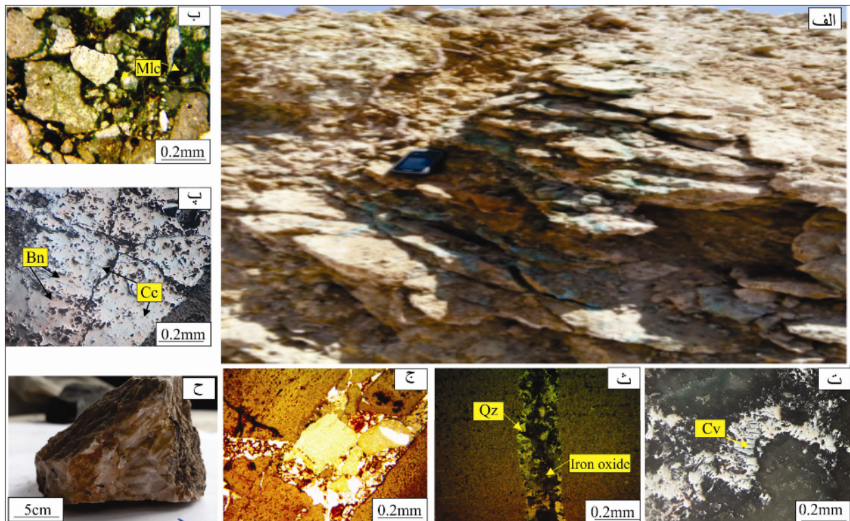
شکل ۴ تصاویر صحرایی و میکروسکوپی از کانی‌سازی منطقه اکتشافی مس مشکان: الف) نمای از رگه مالاکیت، ب) کانی‌سازی مالاکیت در بین قطعه‌های کنگلومرا در نور قطبیده صفحه‌ای، PPI، پ) بournonite و کالکوسیت در PPL، ت) کالکوسیت‌های ثانویه همراه با کوولیت در PPL، ث) رگچه کوارتز-اکسید آهن در نور قطبیده متقاطع، XPL، ج) اکسید آهن در PPL، ح) نمونه دستی از باریت. =Bn بournonite، =Cc کالکوسیت، =Cv کوولیت، =Mlc مالاکیت و =Qz کوارتز [۱۱].
