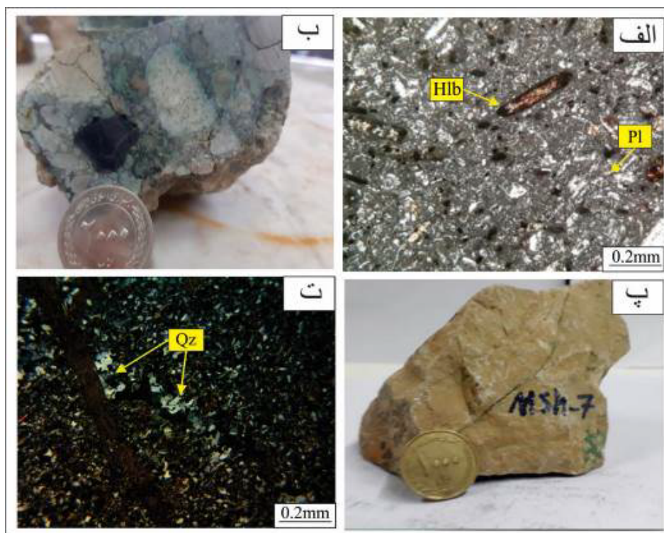
شکل ۳ واحدهای سنگی منطقه مس مشکان: الف) تصویر میکروسکوپی واحد هورنبلند آندزیت، ب) نمونه دستی از کانی‌سازی مالاکیت در بین قطعه‌های کنگلومرا، پ) واحد آهکی و ت) تصویر میکروسکوپی رگچه کوارتز در واحد ماسه‌سنگ. تصاویر میکروسکوپی در نور قطبیده متقاطع، XPL گرفته شده‌اند. Hbl=هورنبلند، Pl=پلاژیوکلاز و Qz=کوارتز (۱۱).
