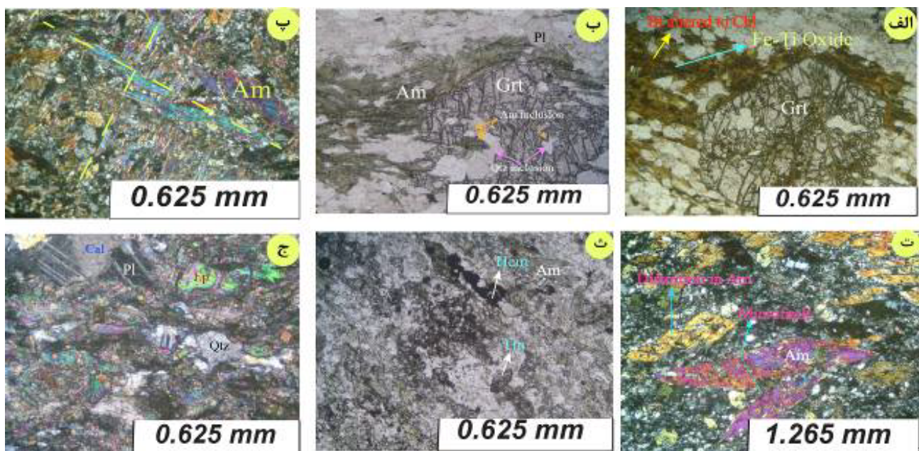
شکل ۳ گارنت آمفیبولیت شامل: الف) همزیستی گارنت و بیوتیت که بیوتیت در فاز پسرودگی به کلریت تجزیه شده است. اکسیدهای Fe-Ti در راستای رخ‌ها و لبه‌های بیوتیت آزاد شده‌اند. گارنت دارای شکستگی‌های لانه زنبوری و نیز پسا زمین‌ساخت است. ب) همزیستی گارنت و آمفیبول کلسیمی که میانبارهایی کوارتز دارای بقایایی از آمفیبول هستند. آمفیبولیت بدون گارنت شامل: پ) دو دسته آمفیبول که به صورت متقاطع و نسبت به هم تصادفی قرار گرفته‌اند. ت) اعوجاج و ریزگسل در آمفیبول. ث) تیتانیت و هماتیت در کنار آمفیبول. ج) شیست‌های اپیدوت-دار که پلاژیوکلاز با ماکل دگرشکلی، کلسیت و اپیدوت در آن مشخص است.
