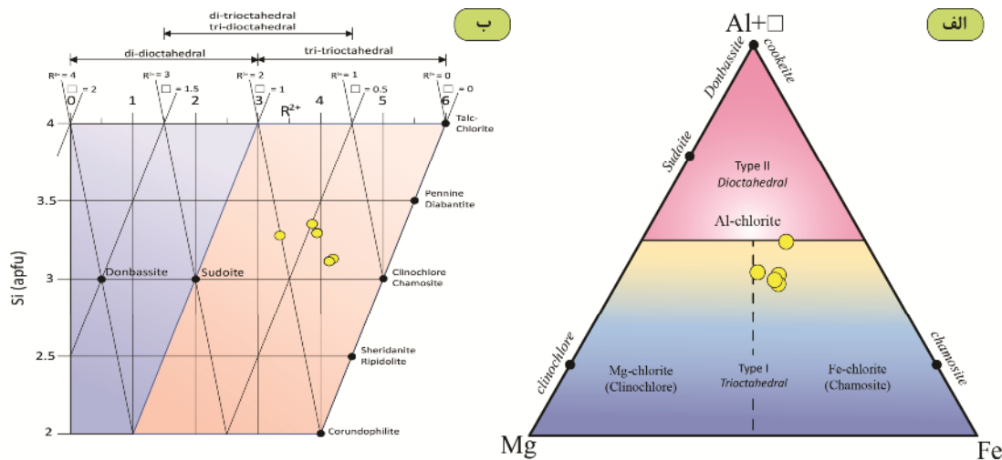
شکل ۷ الف) نمودار Mg-Fe-(Al+□) که براساس آن نمونه‌های کلریت گیسور در گروه I قرار دارند (برگرفته از مرجع [۳۴]). ب) نمودار - که با توجه به آن، نمونه‌های کلریت گیسور در زیرگروه سه-سه هشت وجهی قرار دارند (برگرفته از مرجع [۳۶]).
