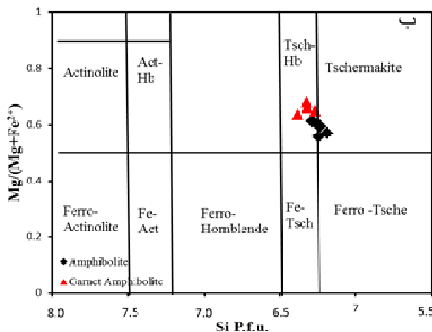
شکل ۵ الف) رده‌بندی آمفیبول‌های موجود در نمونه‌های آمفیبولیت و گارنت آمفیبولیت بر اساس نمودار مرجع [۲۰] که همه نمونه‌ها در گستره آمفیبول‌های کلسیمی قرار گرفته‌اند و ب) جایگاه ترکیبی آمفیبول‌ها در آمفیبولیت‌ها و گارنت آمفیبولیت‌های منطقه گل‌گهر، بر اساس نمودار تقسیم‌بندی آمفیبول‌های کلسیمی از مرجع [۲۰].
