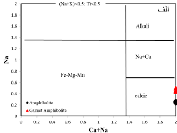
شکل ۵ الف) رده‌بندی آمفیبول‌های موجود در نمونه‌های آمفیبولیت و گارنت آمفیبولیت بر اساس نمودار مرجع [۲۰] که همه نمونه‌ها در گستره آمفیبول‌های کلسیمی قرار گرفته‌اند و ب) جایگاه ترکیبی آمفیبول‌ها در آمفیبولیت‌ها و گارنت آمفیبولیت‌های منطقه گل‌گهر، بر اساس نمودار تقسیم‌بندی آمفیبول‌های کلسیمی از مرجع [۲۰].
