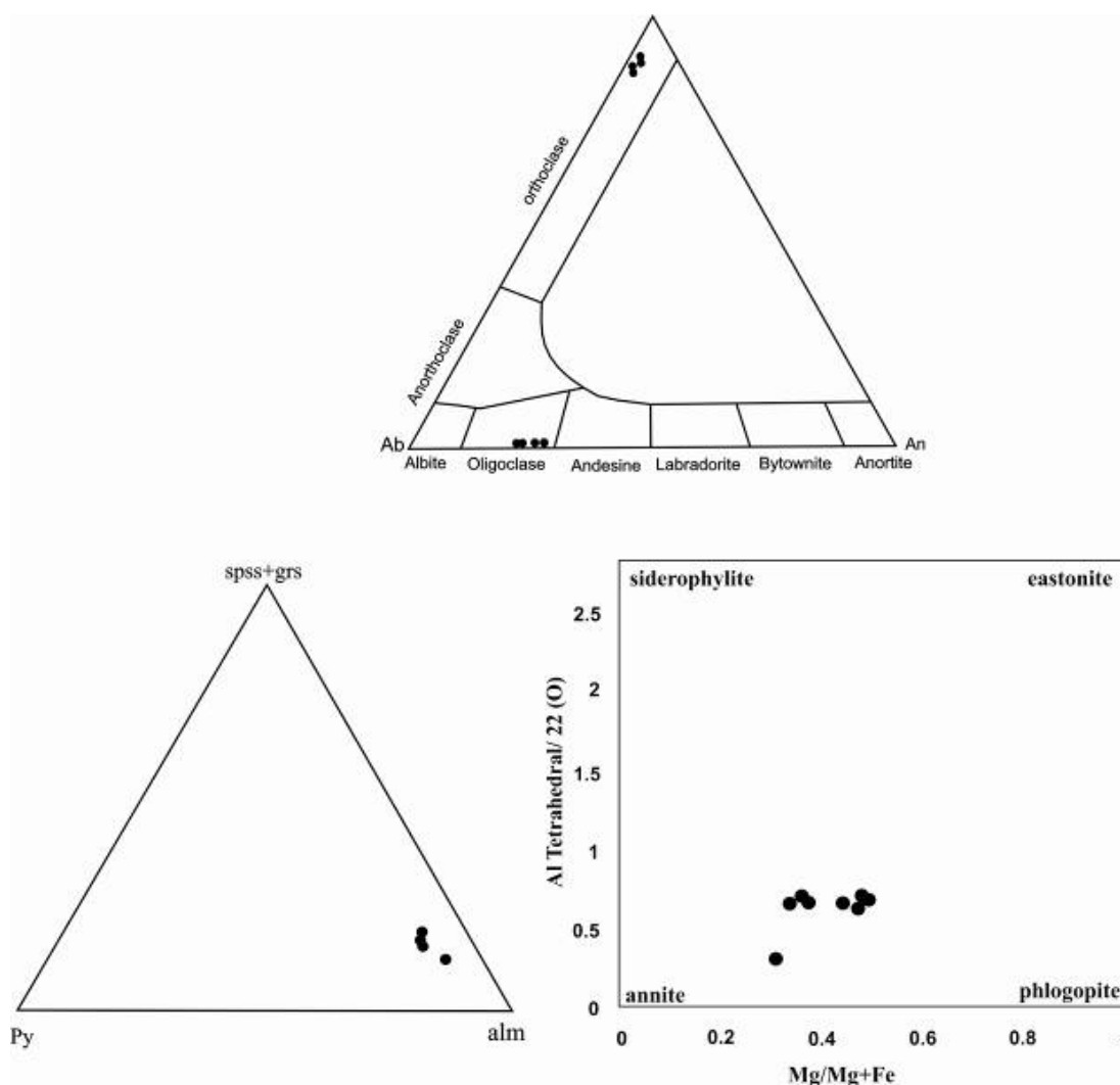
شکل ۵ ترکیب شیمیایی کانی‌ها در میگماتیت‌های بروجرد: الف) ترکیب شیمیایی پلاژیوکلازها و فلدسپارهای قلیایی در نمودارهای سه تایی Ab, Or, An [۲۶]، ب) ترکیب شیمیایی گارنت نمودار سه تایی Fe, Mg, Mn+Ca [۲۷] و پ) ترکیب شیمیایی بیوتیت‌ها در نمودار Mg/Mg+Fe نسبت به Al\ Tetrahedral/22(O) چاروچی که بین قطب فلوگوپیت و آنیت قرار گرفته‌اند
