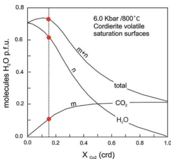
شکل ۸ نمودار تعیین تعداد مولکول‌های آب و CO_2 موجود در شبکه کردیریت [۳۵].
