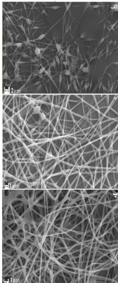
شکل ۵ تصویر SEM الیاف الکتروپسپس شده با پلیمر PVA با غلظت الف (۵٪ وزنی ب) ۷٪ وزنی و پ (۵٪ درصد وزنی).
