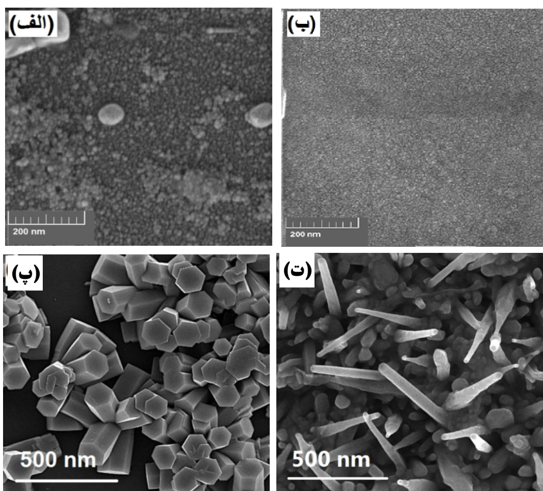
شکل ۳ تصاویر FESEM لایه‌ی بذر نمونه‌ی (الف) نمونه‌ی (ب) و نانومیله‌های اکسید روی با غلظت محلول ۲۵ mM رشد یافته بر لایه‌ی بذر نمونه‌ی الف، پ) نمونه‌ی ب (ت).
