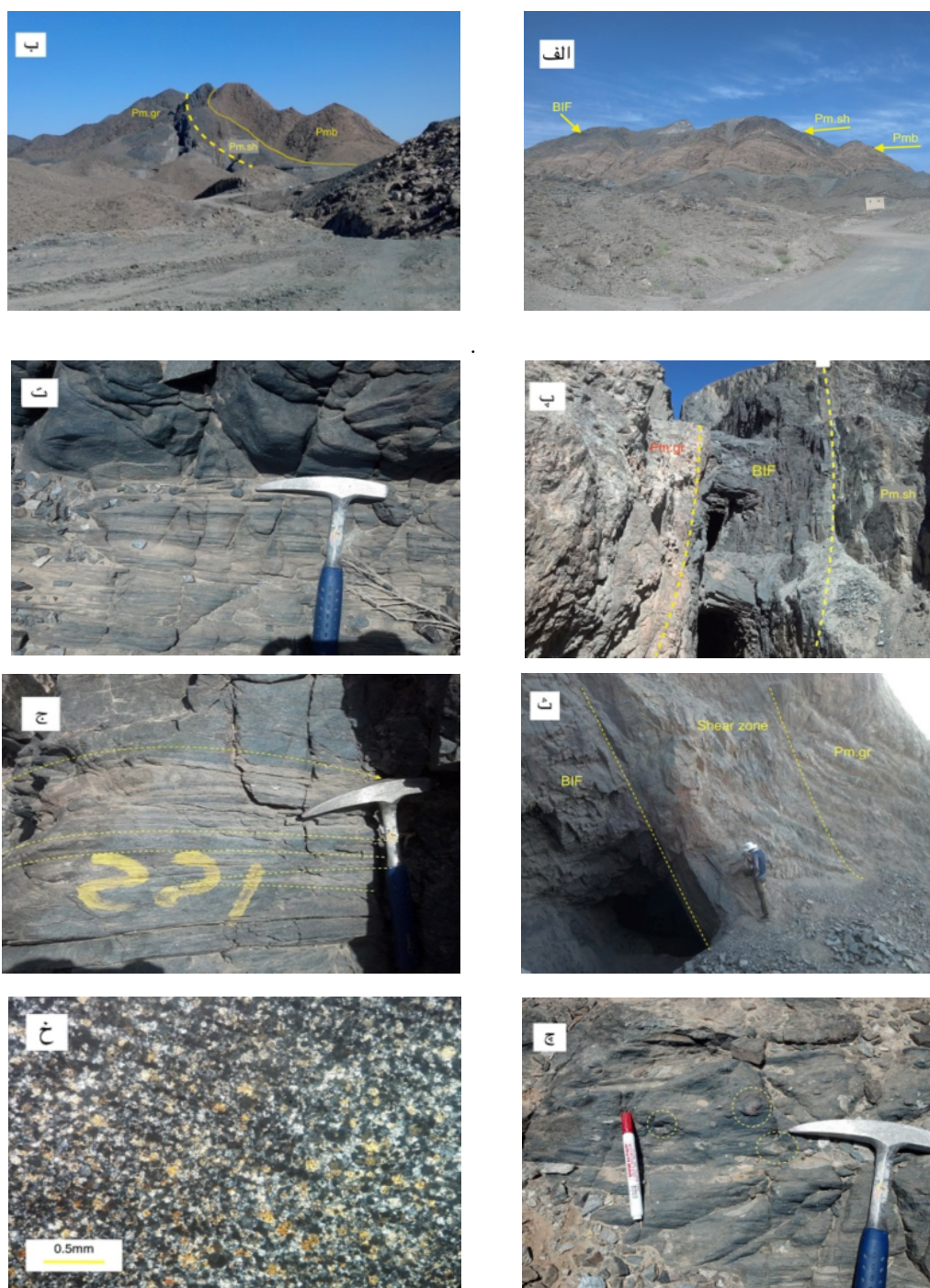
شکل ۴ الف: رخنمون اصلی و سیما ساز واحد کربناتی و واحد موسکوویت شیست که با مجموعه‌ی دگرگونی زیرین مرزی گسلی دارند (دید به سمت شمال غرب)، ب: رخنمون واحد کربناتی و موسکوویت شیست‌ها که به‌صورت برگشته با واحد گرانیت‌های - قلیایی میلوئیتی شده مرزی گسلی دارند، (دید به سمت شرق)، پ: نوار کانه‌زایی اصلی به صورت همشیب و پیوسته با واحد موسکوویت شیست و مرز گسله و میلوئیتی با واحد گرانیت‌های قلیایی میلوئیتی شده (دید به سمت شرق)، ت: مرز واحد موسکوویت شیست با نوار کانه‌زایی اصلی و ادامه تناوب نازک لایه‌های هماتی درون واحد موسکوویت شیست، ث: مرز گسله و متورق (زون برشی) نوار کانه‌زایی اصلی با گرانیت‌های میلوئیتی شده (دید به سمت غرب)، ج: لایه‌ها و عدسی‌های شیستی و سنگ‌های رسوبی دگرگون شده، بین نوار کانه‌زایی اصلی و کانسنگ هماتی، چ: قطعات و سنگ‌های بیگانه درون نوار کانه‌زایی اصلی، خ: تصویر میکروسکوپی قطعات بیگانه بین کانسنگ هماتی نوار کانه‌زایی اصلی که تماماً از ذرات به هم فشرده کوارتز و کانی‌های کدر با حاشیه مضرسی تشکیل شده‌اند (XPL، درشت‌نمایی 50X)، (Pph: واحد اسلیت و فلیت، Pm.sh: واحد موسکوویت - شیست، Pm.gr: واحد گرانیت میلوئیتی شده، Pmb: واحد کربناته).
