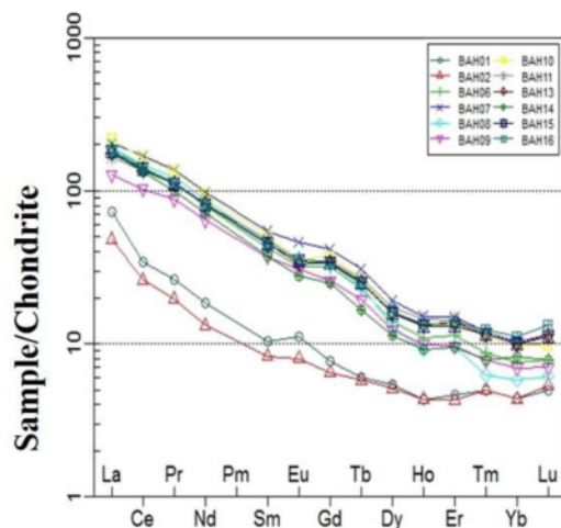
شکل ۱۰ الف) الگوی تغییرات جرم REEها طی کائولینیتی‌شدن سنگ‌های داسیتی در بهاریه. ب) الگوی توزیع REE ها بهنجار شده به کندریت [۱۵] در نمونه‌های کائولن و سنگ‌های داسیتی بهاریه.
