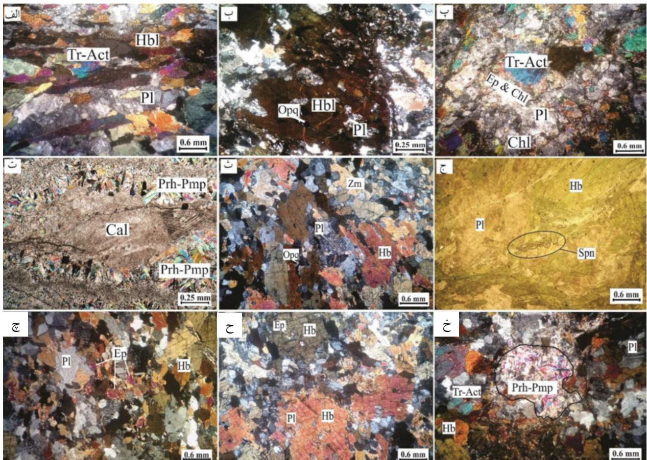
شکل ۲ تصاویر میکروسکوپی پارآمفیبولیت و ارتو-آمفیبولیت: الف- پلاژیوکلاز و آمفیبول با بافت ناماتوبلاستیک در پارآمفیبولیت، ب- میانبار-های پلاژیوکلاز در درون هورنبلند در پارآمفیبولیت، پ- تبدیل هورنبلند به اپیدوت، کلریت و ترمولیت- اکتینولیت طی دگرگونی پسروده در شرایط رخساره‌ی شیبست سبز، ت- فراوانی کلسیت به همراه رگه‌های پره‌نیت- پمپلئیت در پارآمفیبولیت‌ها، ث- فراوانی هورنبلند با بلورهای شکل‌دار تا نیمه‌شکل‌دار و کانی پلاژیوکلاز با ماکل تکراری در ارتوآمفیبولیت، ج- اسفن در ارتوآمفیبولیت، چ- کانی اپیدوت حاصل از دگرگونی پسروده در ارتوآمفیبولیت، ح: میانبارهای کانی اپیدوت و پلاژیوکلاز درون هورنبلند در ارتوآمفیبولیت و خ- جانیشینی پره‌نیت- پمپلئیت به جای پلاژیوکلاز در ارتوآمفیبولیت. (Pl): پلاژیوکلاز، (Hb): هورنبلند، (Tr): ترمولیت، (Act): اکتینولیت، (Opq): کانی کدر، (Ep): اپیدوت، (Chl): کلریت، (Cal): کلسیت، (Prh-Pmp): پره‌نیت- پمپلئیت، (Zrn): زیرکن، (Spn): اسفن [۸]، (تصویر ج در نور قطبیده صفحه‌ای PPL، و سایر تصاویر در نور قطبیده متقاطع، XPL، ثبت شده‌اند).
