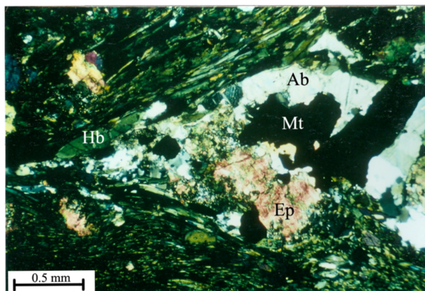
شکل ۶ تصویر میکروسکوپی از هورنبلندی با بافت جریان‌ی کانسار باباعلی، نمونه‌ی 38/B1H، عمق ۳۸ متری.
