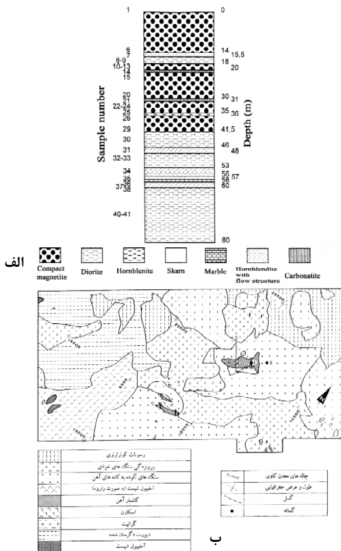
شکل ۳ الف) نیمرخ گمانه‌ی حفاری بااعلی ب) موقعیت چاله‌های معدن کاوی در نقشه‌ی زمین‌شناسی کانسار بااعلی [۱۰].
