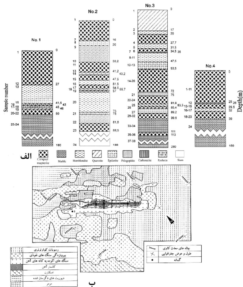
شکل ۲ الف) نیم‌رخ گمانه‌های ۱، ۲، ۳ و ۴ (ب) موقعیت چاله‌های معدن کاوی در نقشه‌ی زمین‌شناسی کانسار گلالی [۱۰] (با تغییرات).
