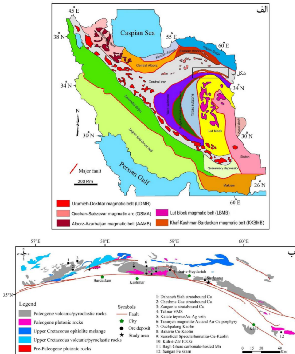
شکل ۱ الف) تقسیم‌بندی پهنه‌های ساختاری-رسوبی ایران (برگرفته از مرجع [۱۷] با تغییرات)، ب) نقشه ساده شده کمربند ماگمایی خواف-کاشمر-بردسکن همراه با کانی‌سازی‌های مهم و جایگاه منطقه مورد بررسی.
