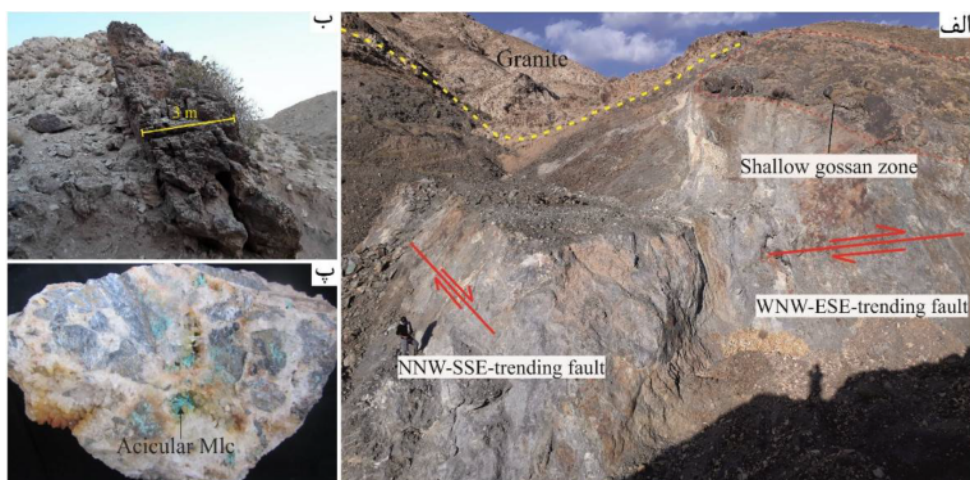
شکل ۵ الف) محل تلاقی دو گسل راستالغز میزبان رگه سیلیسی-سولفیدی در واحد شمشک (دید به سمت شمال)، ب) رگه سیلیسی-سولفیدی سبتر (دید به سمت شمال)، پ) برش به هم ریخته غنی از سیمان و حضور کوارتز با بافت شانه‌ای و ملاکیت سوزنی به عنوان سیمان قطعه‌ها.
