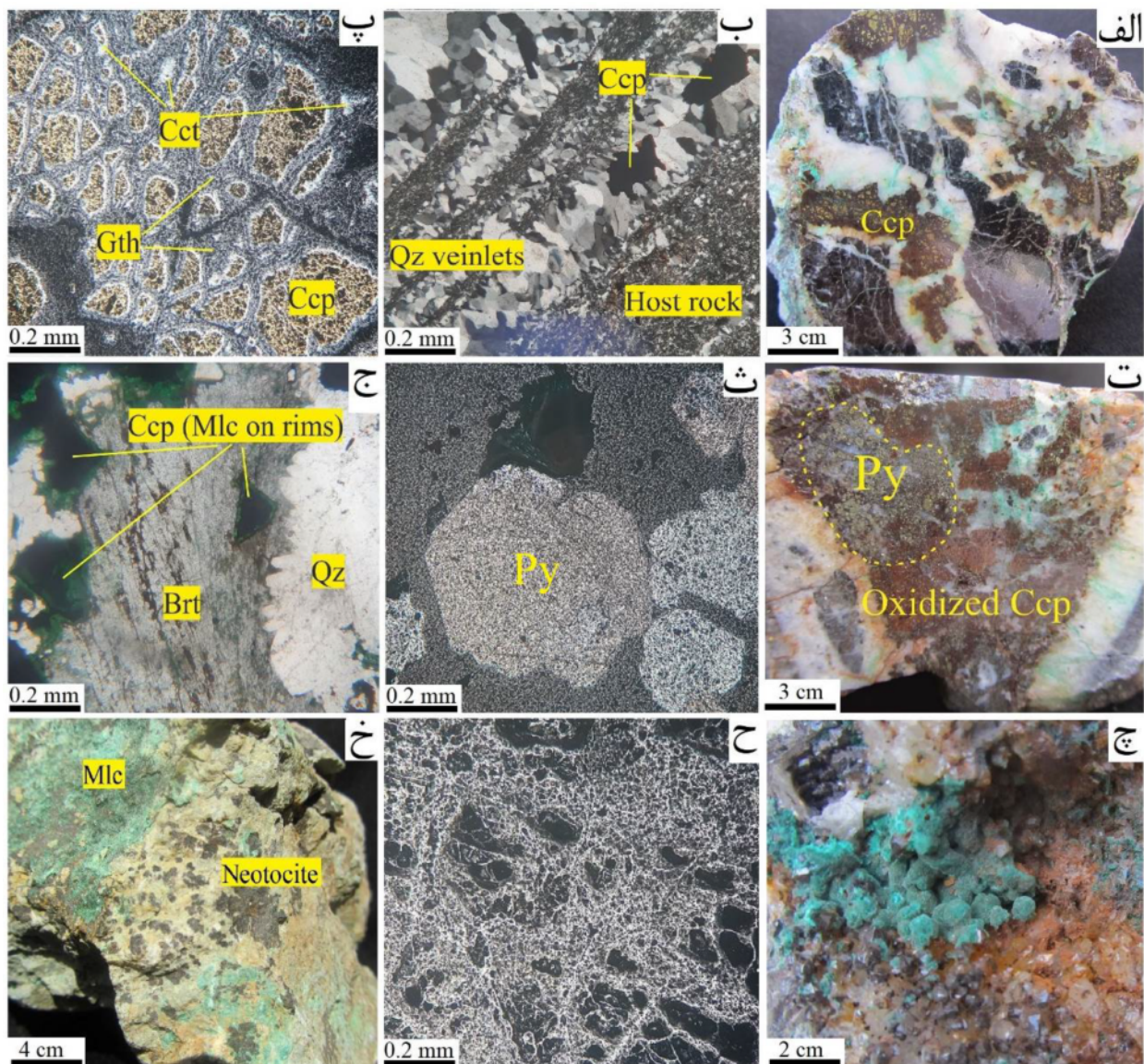
شکل ۶ الف) نمونه دستی کالکوپیریت-کوارتز در رگه سیلیسی برشی شده، ب) بافت پرکننده فضای خالی کوارتز همراه کالکوپیریت، نور قطبیده متقاطع، (پ) بافت جانیشینی ثانویه کالکوسیت و گوتیت در نتیجه اکسید شدن کالکوپیریت، نور قطبیده صفحه ای، (PPL)، ت) نمونه دستی پیریت و کالکوپیریت در حال تبدیل شدن به اکسیدهای آهن در رگه سیلیسی برشی شده، ث) پیریت خودشکل، (PPL)، ج) رگچه کوارتز-کالکوپیریت (در حال تبدیل شدن به مالاکیت) و تشکیل باریت تاخیری دسته‌جاری در فضای خالی (PPL)، چ) مالاکیت با بافت خوشه‌انگوری روی بلورهای کوارتز، ح) بافت جعبه‌ای-اسفنجی در اکسیدهای آهن (PPL)، خ) نئوتوسیت لکه‌ای همراه مالاکیت (Ccp): کالکوپیریت، Py: پیریت، Gth: گوتیت، Cct: کالکوسیت، Mlc: مالاکیت، Brt: باریت، Qz: کوارتز [۲۵].
