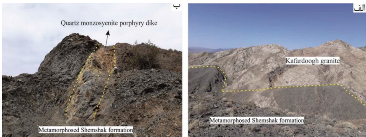
شکل ۳ الف) دورنمایی از توده گرانیتی کافردوغ که به درون سازند شمشک نفوذ کرده است (دید به سمت غرب)، ب) نفوذ دایک مونزوسینیت پورفیری درون سازند شمشک (دید به سمت شمال غرب)
