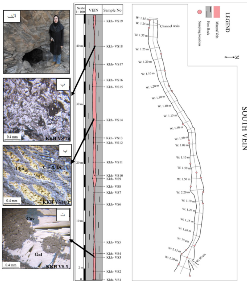
شکل ۵ نیمرخ طولی تونل حفر شده در رگه‌ی جنوبی (مختصات جغرافیای "۵۱° ۲۶' ۵۹" X, "۱۶' ۱۲' ۳۶" Y) و موقعیت نمونه‌های اخذ شده. الف: نما از دهانه‌ی ورودی تونل، ب: نمونه‌ی KKH-VS18 اکسیدهای آهن (هماتیت) در نور XPL. پ: نمونه‌ی 1/ KKH-VS14 رگچه کالکوپیریت در حال تبدیل به کوولیت در نور XPL. ت: نمونه‌ی KKH-VS3 گالن در حال تبدیل شدن به کوولیت و سروزیت (بافت جانشینی) در نور XPL.
