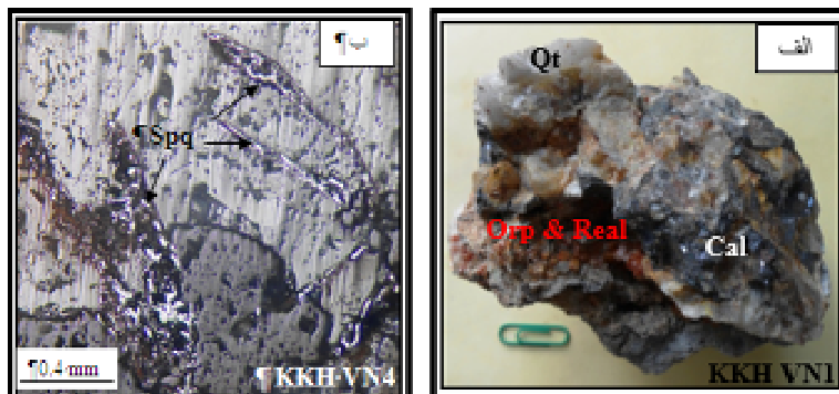
شکل ۶ رخنمون رگه‌ی شمالی؛ دید به سمت جنوب، موقعیت رگه شمالی (مختصات جغرافیای ۳۳ ۲۶ ۵۹ X، ۱۷ ۱۲ ۳۶ Y) و نمونه‌های مورد بررسی. الف: نمونه‌ی KKH-VN1 کانی‌های گالن، کوارتز، اورپیمنت و رالگار در نمونه‌ی دستی. ب: نمونه KKH-VN4 اکسیدهای آهن و کوارتز در مقطع بلوک صیقلی هماتیت (اسپیکیولاریت) با صورت سوزنی و تیغه‌ای.
