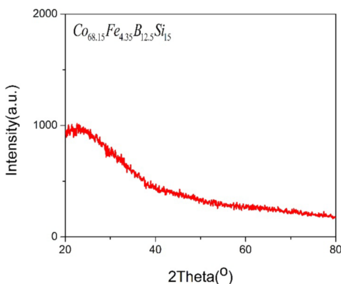
شکل ۲ الگوی پراش پرتو ایکس سیم بی‌شکل کبالت پایه‌ی Co_{68.15}Fe_{4.35}B_{12.5}Si_{15}
