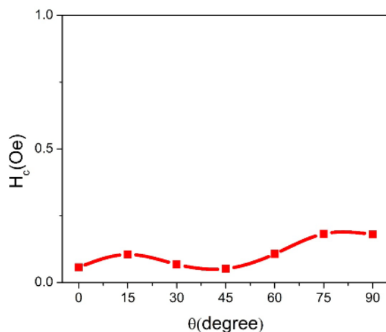
شکل ۶ منحنی میدان وادارندگی بر حسب زاویه برای سیم بی‌شکل کبالت پایه‌ی Co_{0.6815}Fe_{4.35}B_{12.5}Si_5
