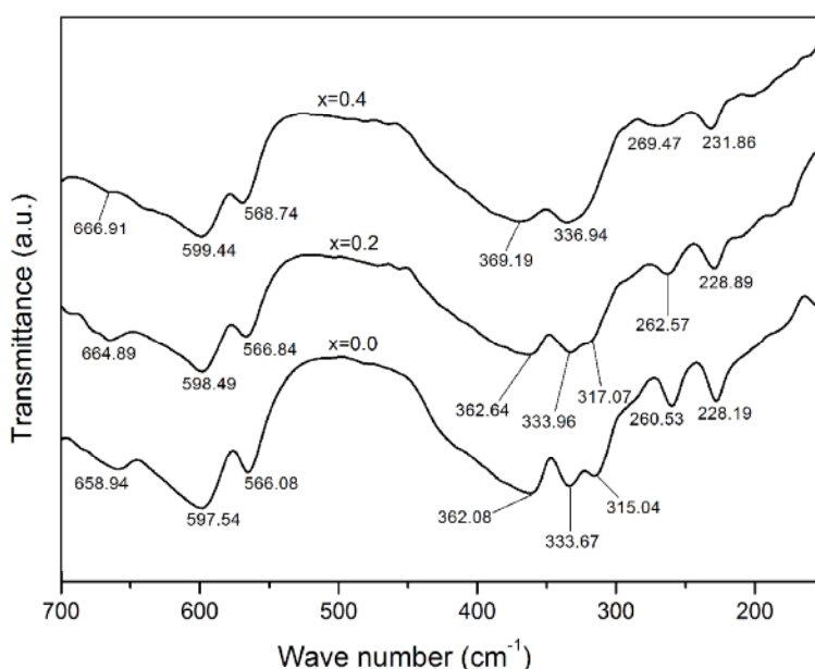
شکل ۳ طیف‌های تبدیل فوریه فروسرخ دور نمونه‌های \text{Y}_3\text{Al}_x\text{Fe}_{5-x}\text{O}_{12} با میزان جانمایی x = (0.0, 0.2, 0.4) .
