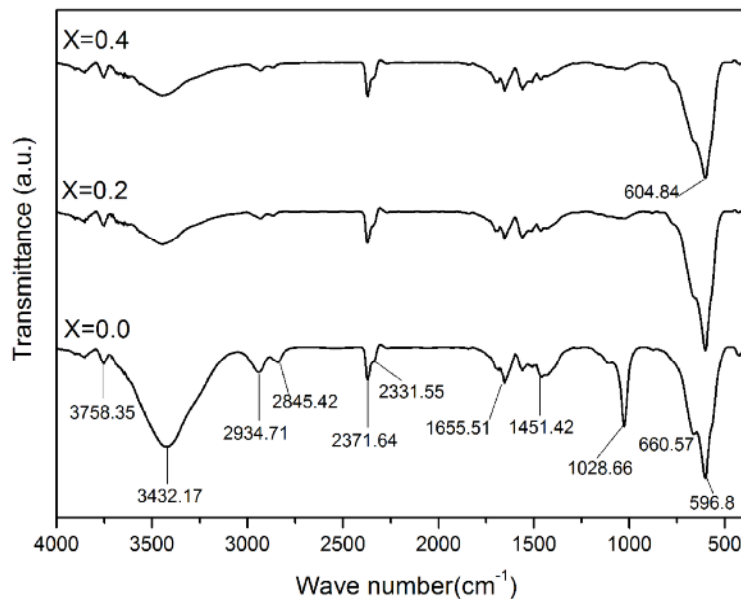
شکل ۴ طیف‌های تبدیل فوریه فرسرخ میانه نمونه‌های Y_3Al_xFe_{5-x}O_{12} با جاننشانی x = (0.0, 0.2, 0.4)
