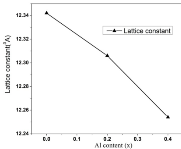
شکل ۲ تغییرات ثابت شبکه و الگوهای پراش پرتو ایکس در بازه‌ی ۳۱-۳۴ درجه‌ی نمونه‌های Y_3Al_xFe_{5-x}O_{12} بر حسب میزان جانمایی x = (0.0, 0.2, 0.4) .
