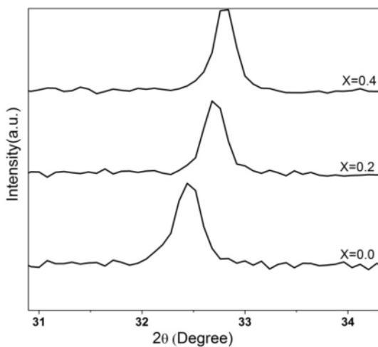
شکل ۲ تغییرات ثابت شبکه و الگوهای پراش پرتو ایکس در بازه‌ی ۳۱-۳۴ درجه‌ی نمونه‌های Y_3Al_xFe_{5-x}O_{12} بر حسب میزان جانمایی x = (0.0, 0.2, 0.4) .
