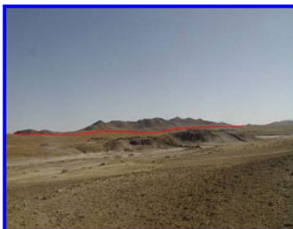
شکل ۴ محدوده توناکار که مرز بین واحدهای کرتاسه و ائوسن Kmlf2 - Esme مشخص شده است (نگاه به سمت جنوب).
