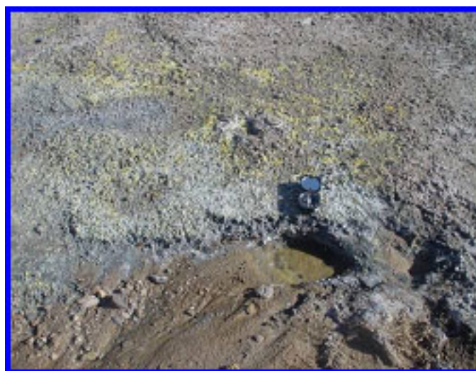
شکل ۵ پراکندگی کانه آلکسیت به همراه گوگرد در رسوب‌ها دیده می‌شود.
