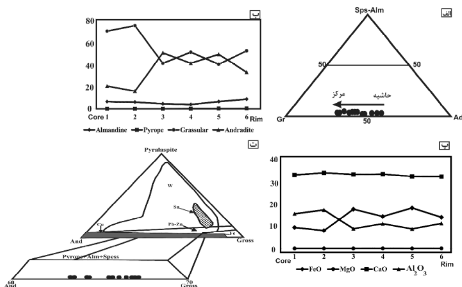
شکل ۴ الف) نمودار سه تایی (اسپسارتین + آلماندن)، (گروسولار) و (آندرادیت) [۸]. ب) نمودار منطقه‌بندی اعضای انتهایی بلور گارنت. پ) نمودار منطقه‌بندی عناصر موجود در بلور گارنت. ت) ترکیب گارنت‌های مورد بررسی در نمودار (Andradite-Grossular-Pyrope+Almandine+Spessartine) برای مقایسه با گارنت‌های اسکارن [۹].
