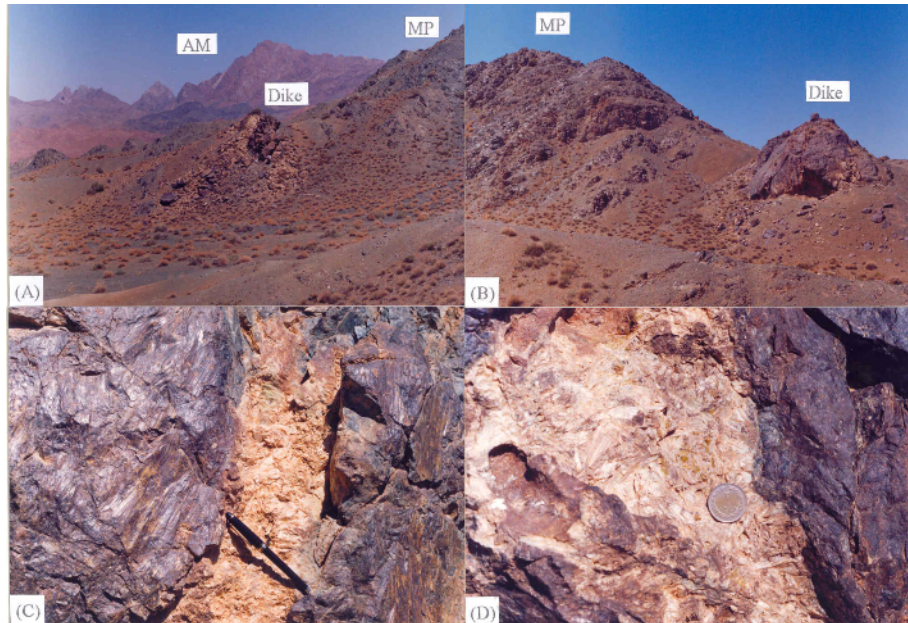
شکل ۳ تصاویر صحرایی رودینگیته‌های موجود در افیولیت شمال انارک (شمال شرق استان اصفهان). (A): دایک رودینگیته شده درون پریدوتیت‌های سرپانتینی شده گوشته (MP)، و دگرگونه‌های انارک (AM) (نگاه به شمال). (B): دایک رودینگیته درون پریدوتیت‌های سرپانتینی شده گوشته، در جنوب شرقی چاه درختک (نگاه به جنوب). (C) و (D): رودینگیته‌های رگه‌ای (بخش روشن) در درون رودینگیته‌های توده‌ای (بخش تیره).
