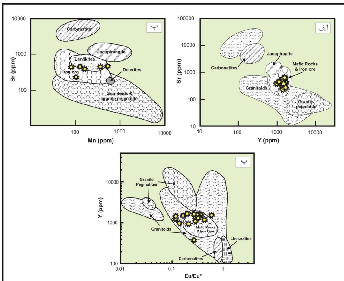
شکل ۱۲ جایگاه نمونه‌های آپاتیت لکه‌سیاه در نمودار الف) Sr - Y، ب) Mn - Sr، و پ) Eu/Eu^* - Y. در همه نمودارها، نمونه‌های مورد بررسی اغلب در گستره مربوط به کانسنگ‌های آهن و سنگ‌های مافیک قرار دارند.
