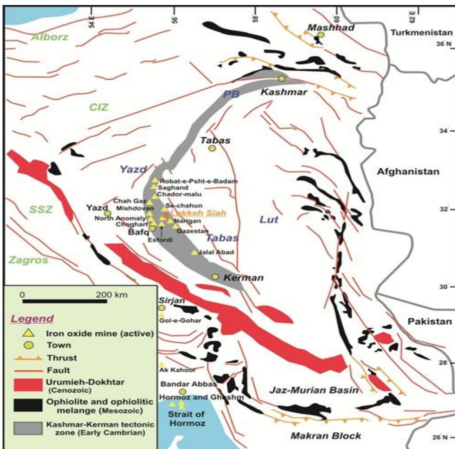
شکل ۱ نقشه ساختاری بخش شرقی- مرکزی ایران و جایگاه پهنه زمین ساختی کاشمر- کرمان و کانسار لکه‌سیاه بر آن [۱۳]. (SSZ: پهنه سندنج- سیرجان، CIZ: پهنه ایران مرکزی و PB: قطعه پشت بادام).
