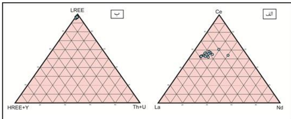
شکل ۶ ترکیب موناژیت‌های لکه‌سیاه در الف) نمودار La-Ce-Nd و ب) نمودار HREE+Y-LREE+Th+U. [۲۸]. جدول ۳ نتایج تجزیه ریزکاو الکترونی کانی موناژیت در کانسار لکه‌سیاه (برحسب درصد وزنی).
